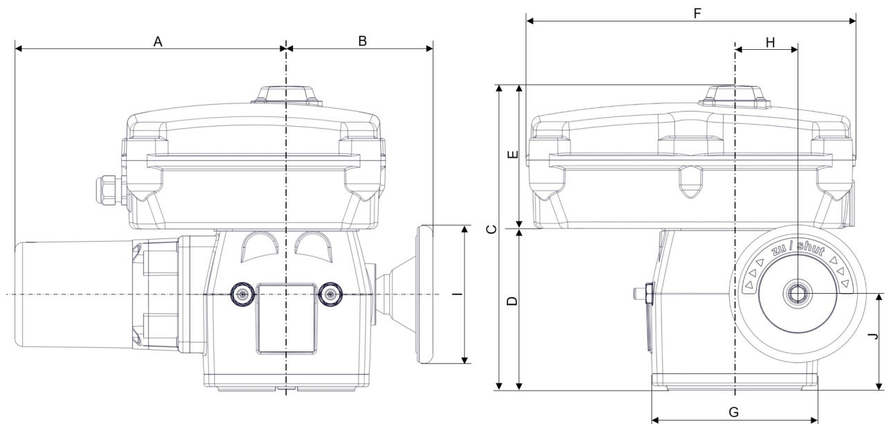
Joonis 3: Mõõtmed
