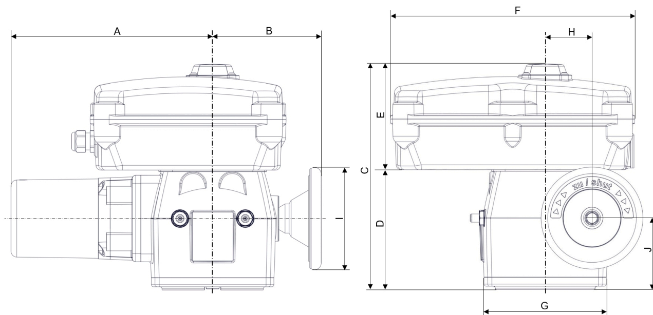
Obr. 3: Rozmery
