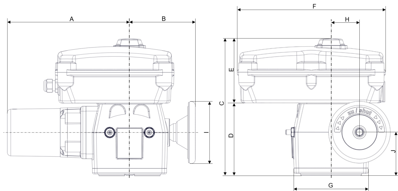
Fig. 3: Dimensiuni
