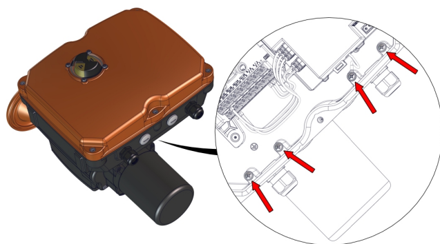
Fig. 13: Racord împământare
