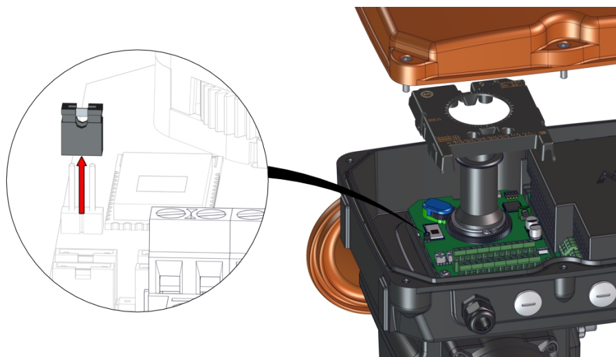
Fig. 15: Mufă de conectare
