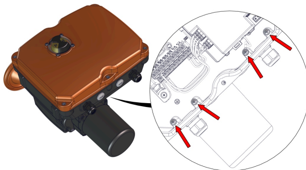
Kuva 13: Suojajohdinliitäntä
