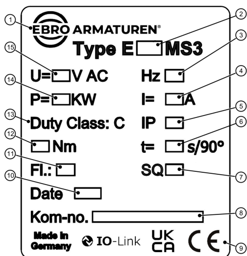
Kuva 1: Tyyppikilpi MS3
