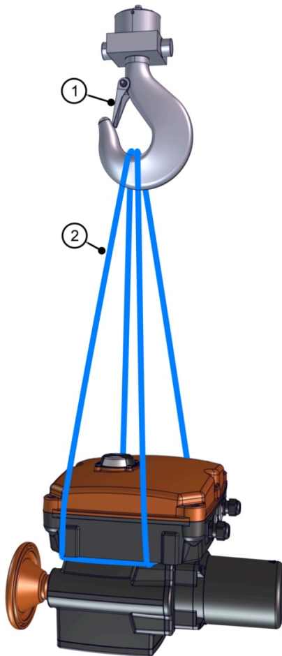
Kuva 5: Säätolaitteen nostaminen
