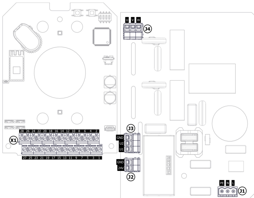
Kuva 7: KytKentäliittimet
