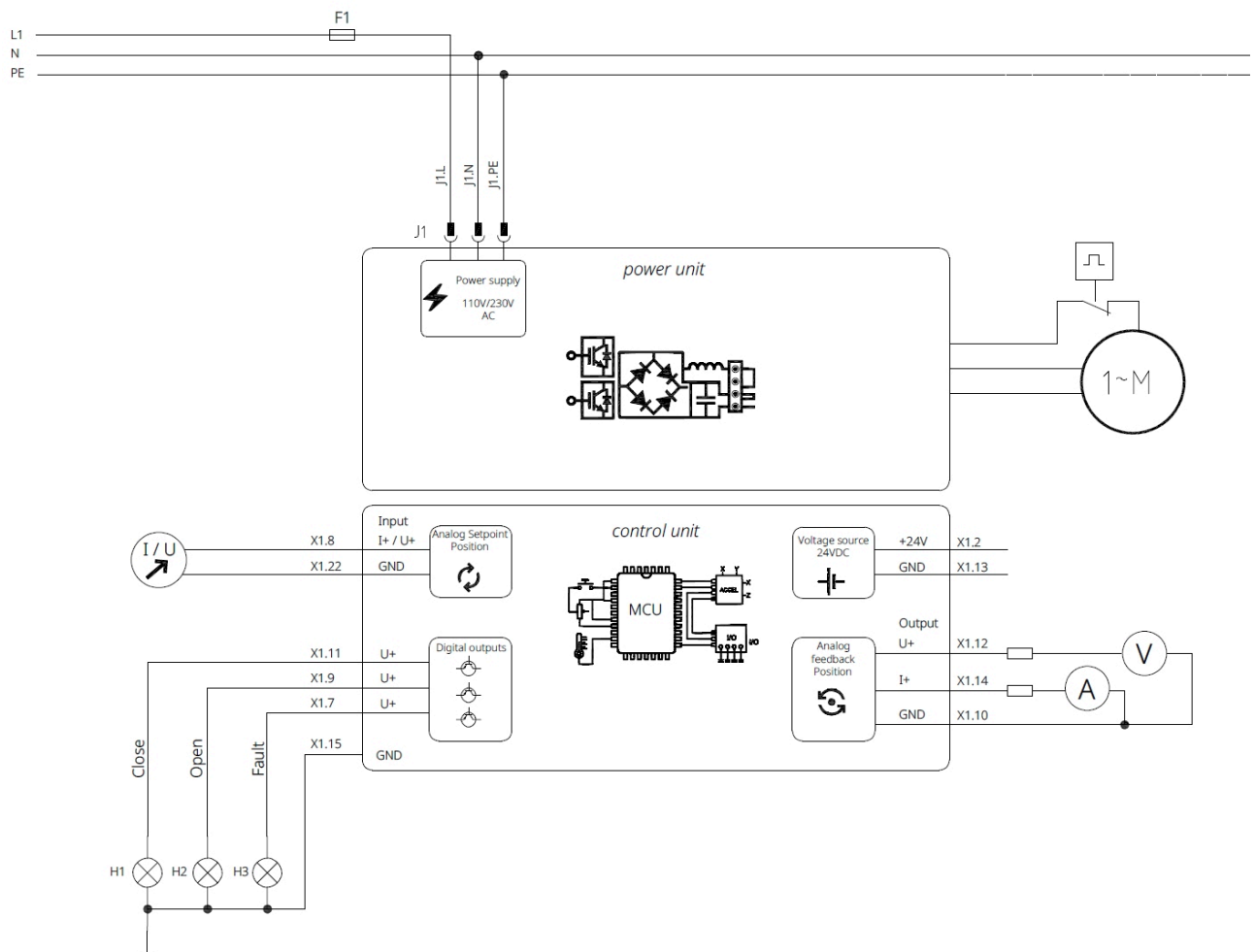
Фиг. 10: Предложение за свързване на електрическо управлящо задвижване MS3
