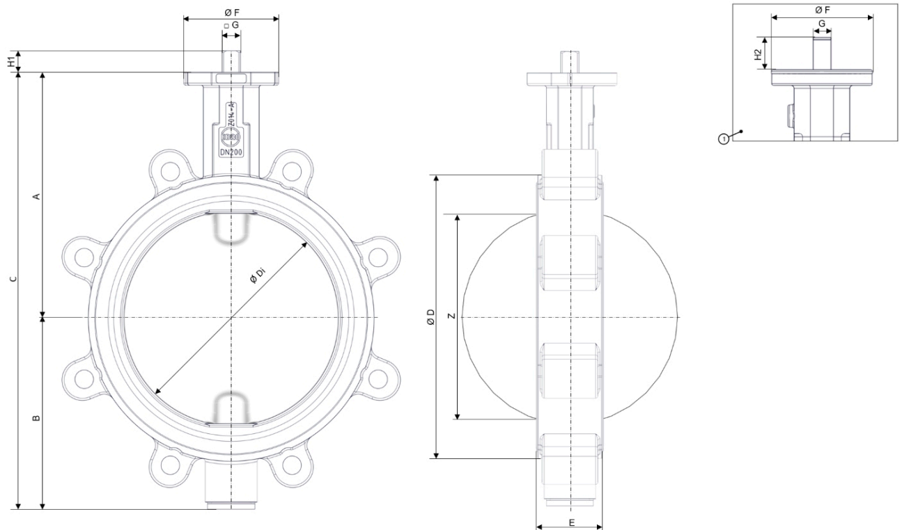
Фиг. 3: Основни размери Z014-B
