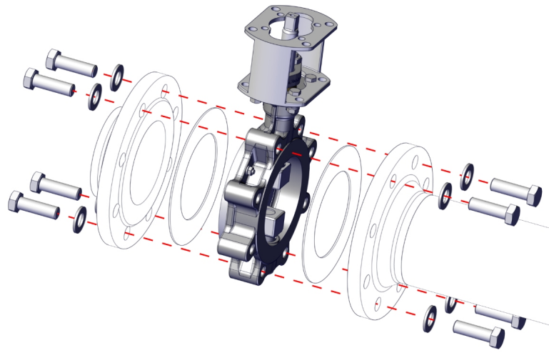
Şek. 8: Flanşlı kapak konumlandırma
