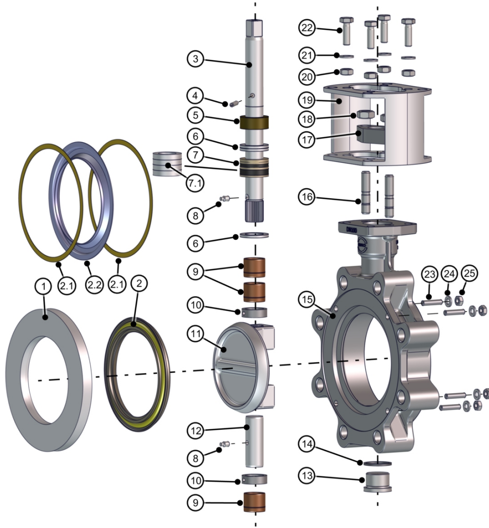
Şek. 15: Parça listesi HP114-HF
