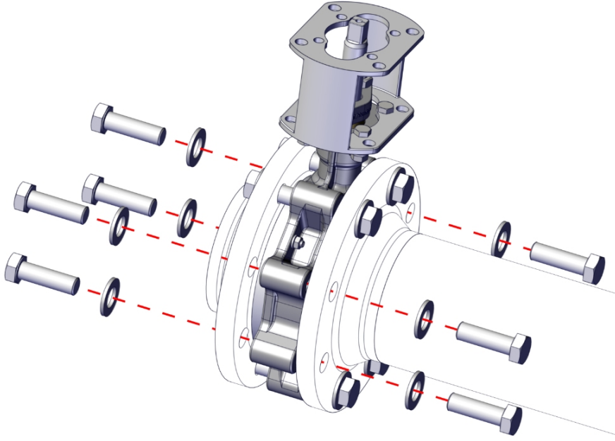
Şek. 9: Flanşlı kapağı vidalama
