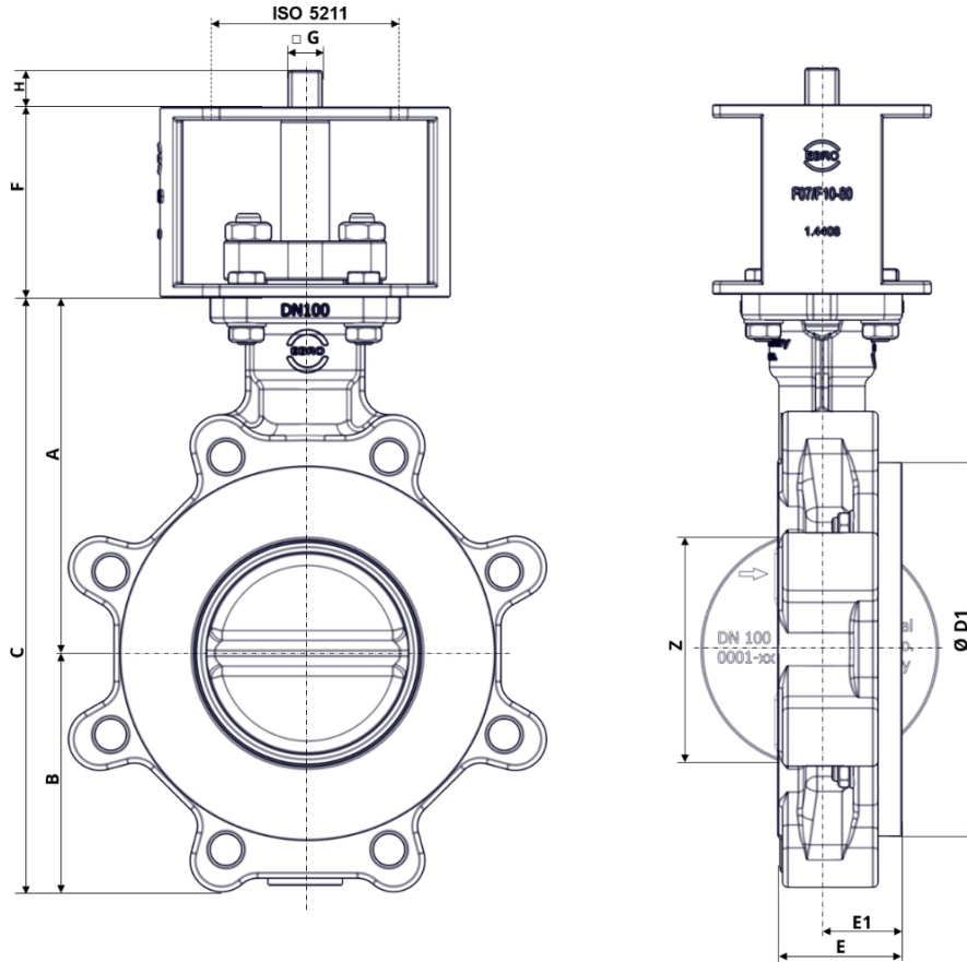
Şek. 3: Ana boyutlar HP114-HF
