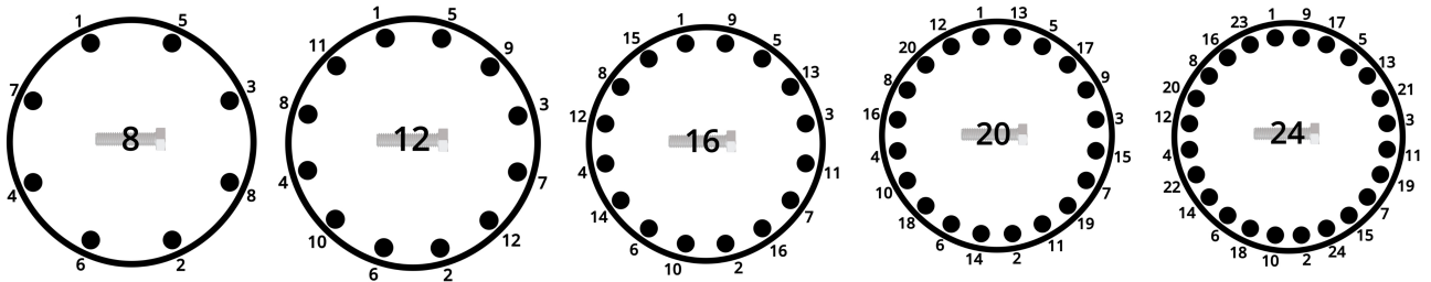
Şek. 12: Boru flanş bağlantılarının sırası
