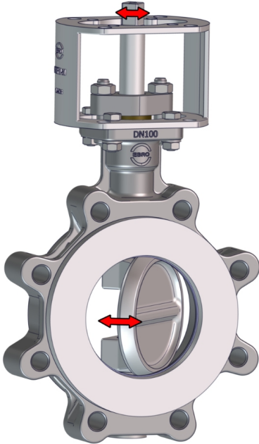
Şek. 4: Hareketli parçalar
