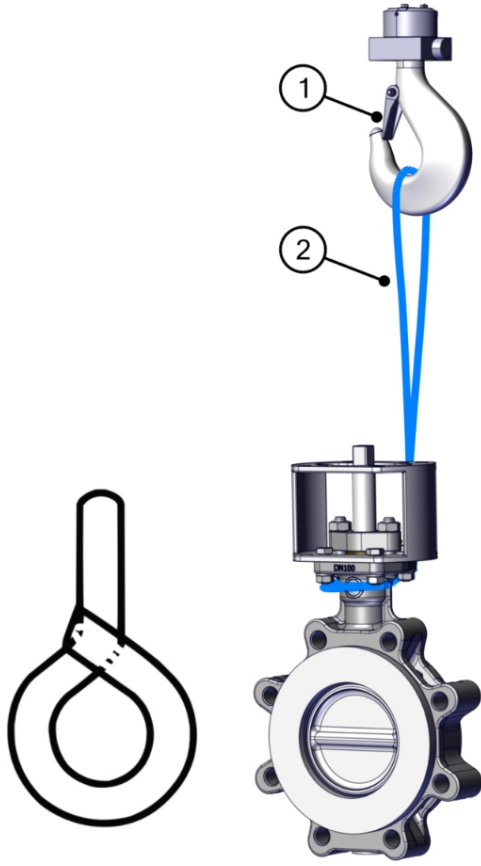
Şek. 6: Flanşlı kapak vinçle kaldırma
