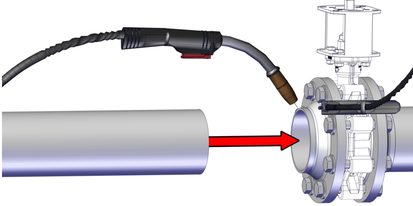
Şek. 10: Boruyu flanşla kaynaklamak
