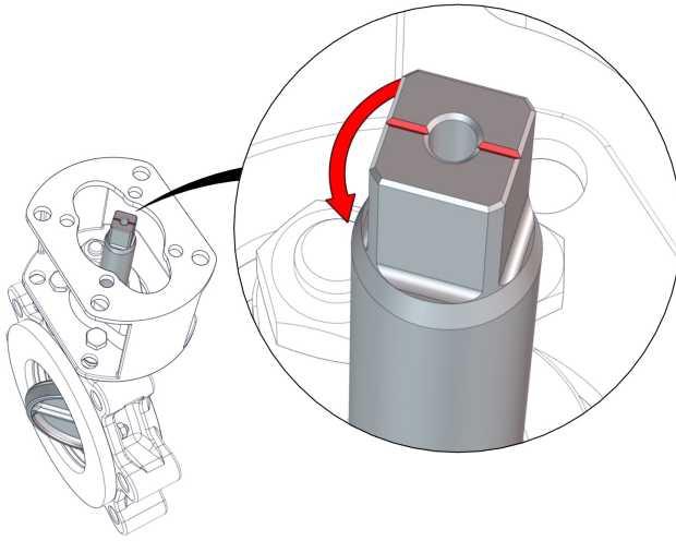
Şek. 14: Çalıştırma yönü
