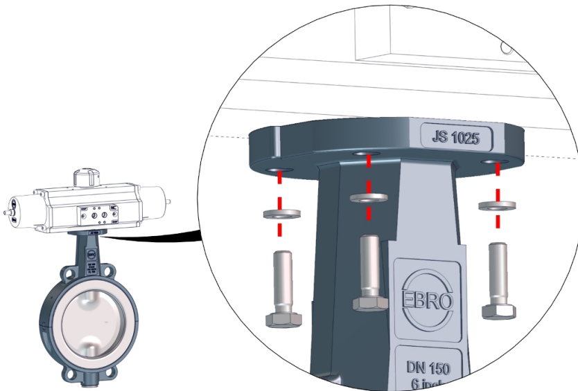
Şek. 7: Prinzip Komponenten montieren
