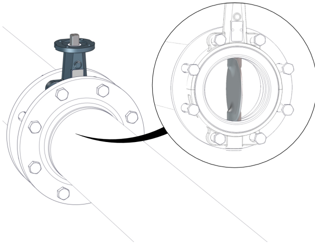
Şek. 13: Rohr spülen
