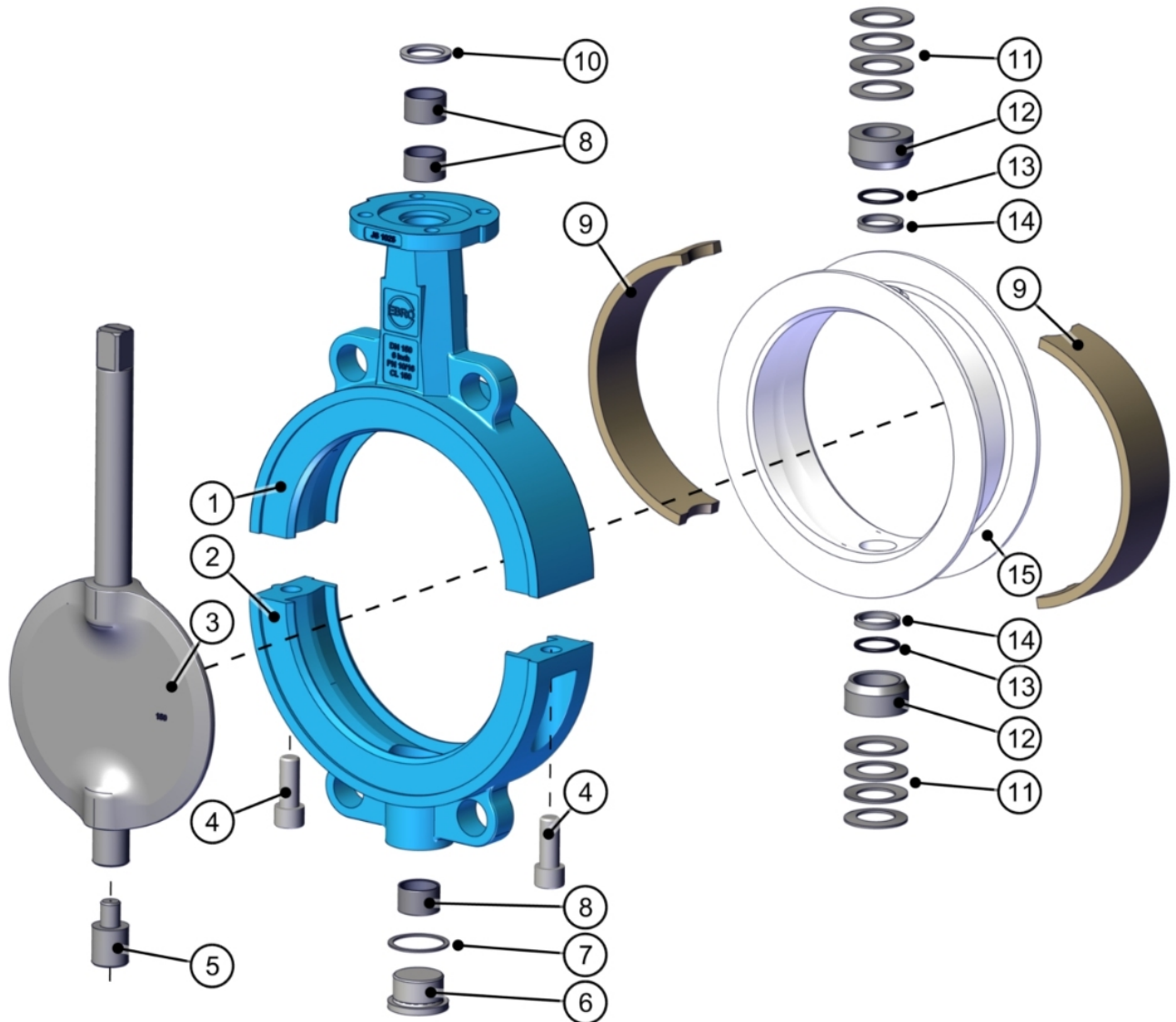
Şek. 16: Stückliste T211-A ab DN40
