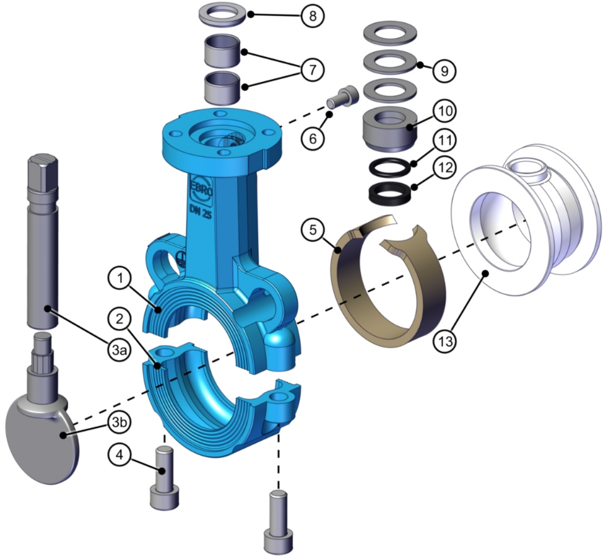
Şek. 15: T211-A Dn32'ye kadar Parça listesi
