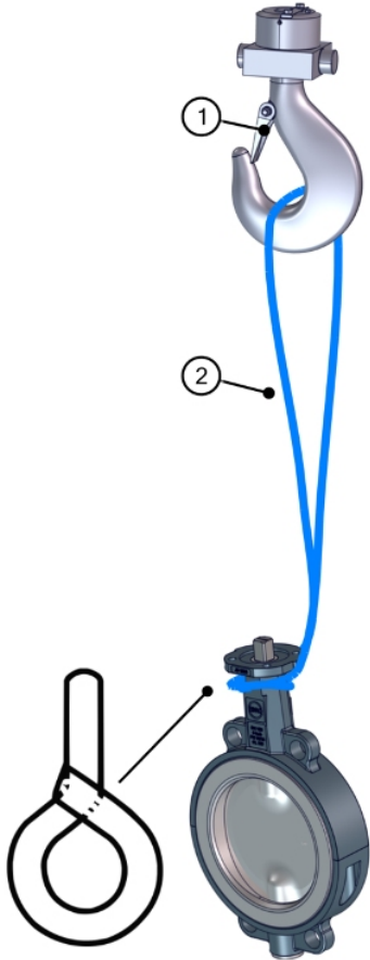
Şek. 6: Zwischenflanschklappe kranen
