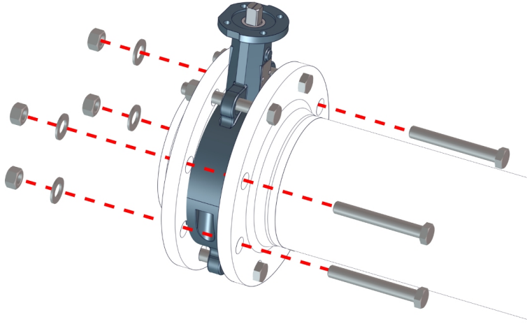
Şek. 9: Zwischenflanschklappe verschrauben
