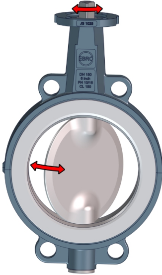
Şek. 4: Hareketli parçalar
