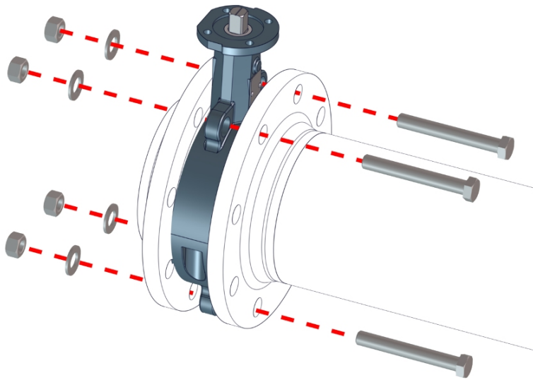
Şek. 8: Zwischenflanschklappe positionieren
