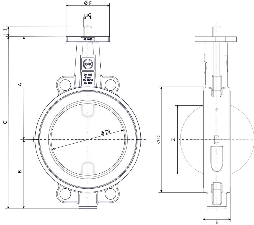
Şek. 3: Ana boyutlar T211-A
