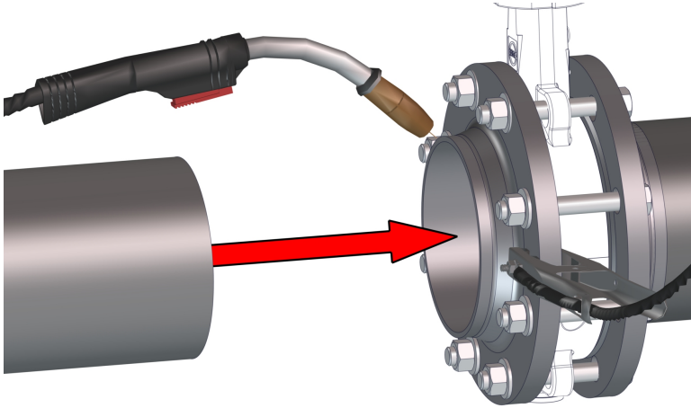
Şek. 10: Rohr mit Flansch verschweißen
