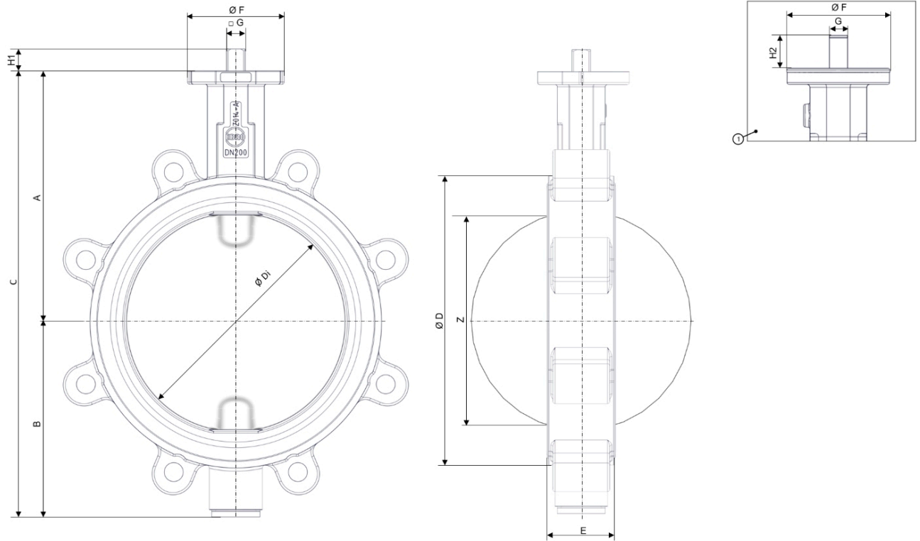
Şek. 3: Ana boyutlar Z014-B
