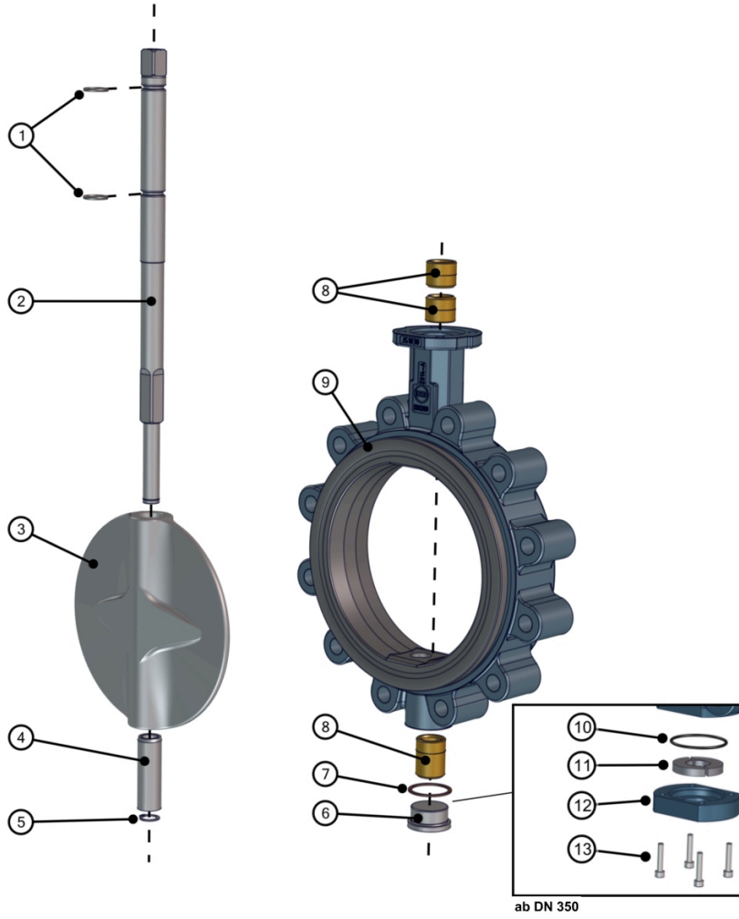
Şek. 16: TS mili parça listesi Z014-B
