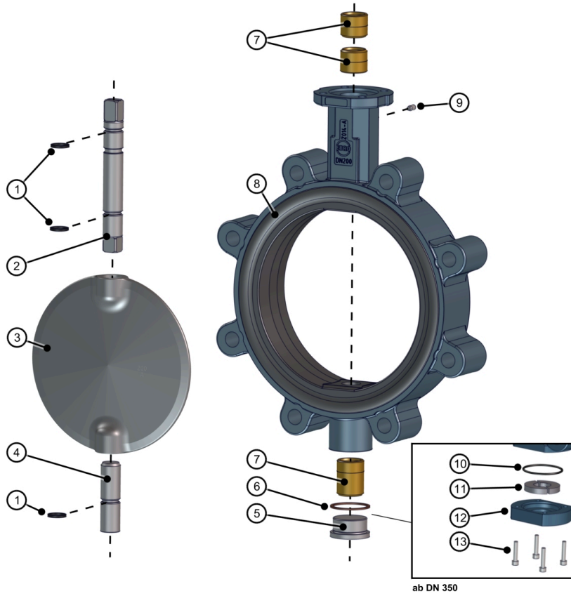
Şek. 15: Parça listesi Z014-B
