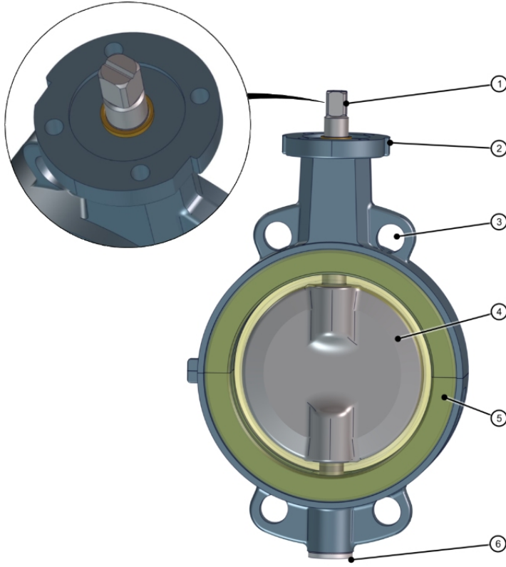
Şek. 2: Bileşenler
