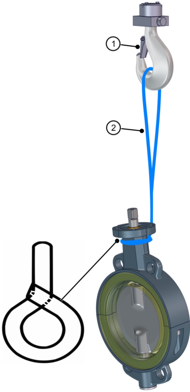
Şek. 6: Ara flanş klapesini vinçle kaldırma
