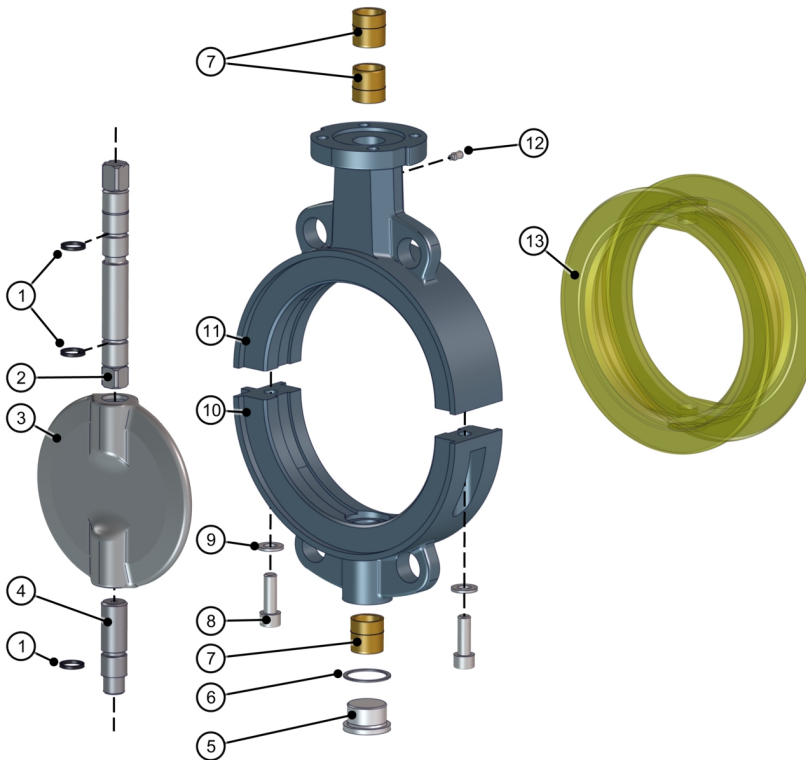
Şek. 15: Parça listesi Z011-GMX
