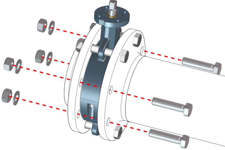
Şek. 9: Ara flanş kapağını vidalama
