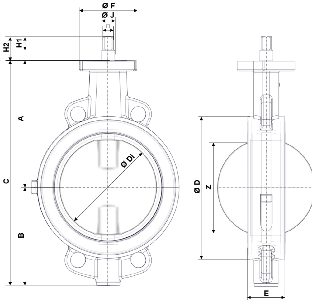
Şek. 3: Ana boyutlar Z011-GMX
