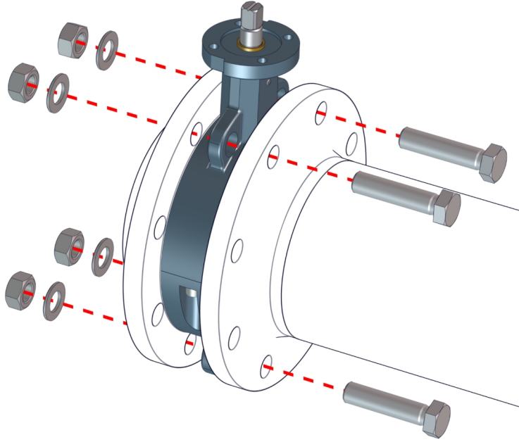
Şek. 8: Ara flanş klapesini konumlandırma
