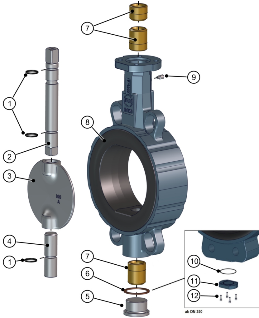
Şek. 15: Bölünmüş mil parça listesi Z011-B
