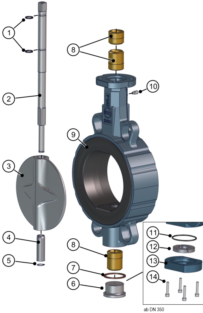
Şek. 16: TS mili parça listesi Z011-B
