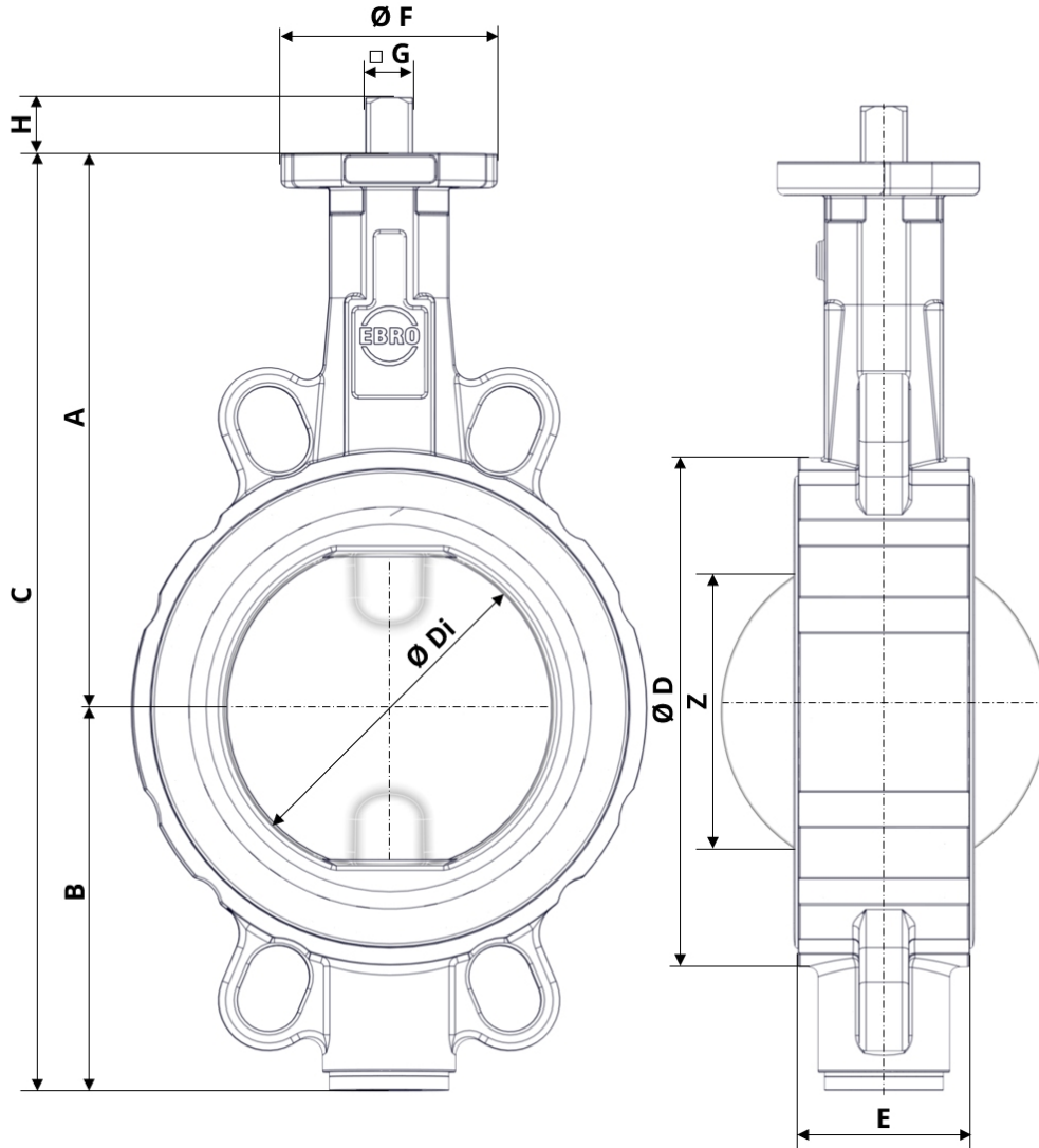
Şek. 3: Ana boyutlar Z011-B
