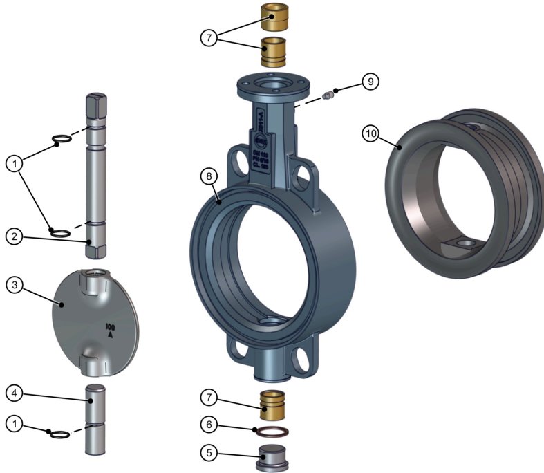
Şek. 15: Parça listesi Z011-AS
