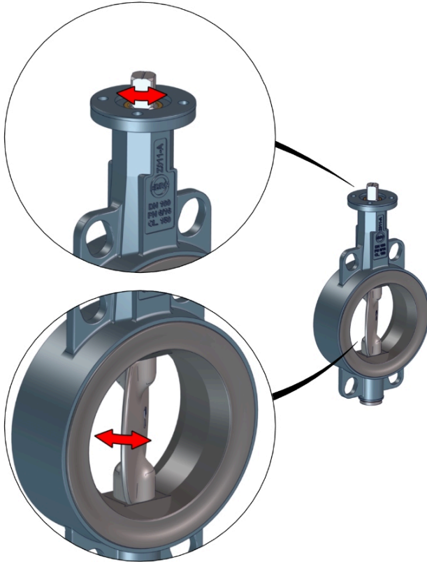
Şek. 4: Hareketli parçalar
