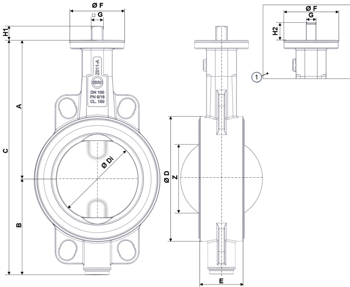
Şek. 3: Ana boyutlar Z011-AS
