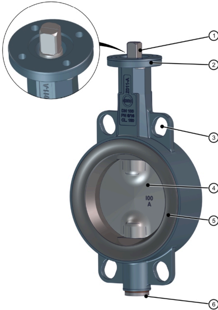
Şek. 2: Bileşenler
