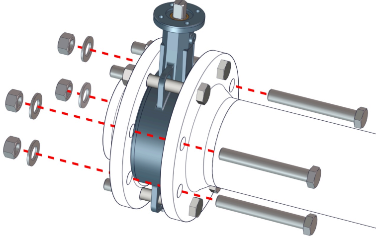
Şek. 9: Ara flanş kapağını vidalama
