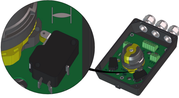
Şek. 9: Kam ayarı "KAPALI"
