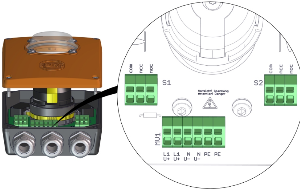
Şek. 6: SBU - Basic konektör şeridi
