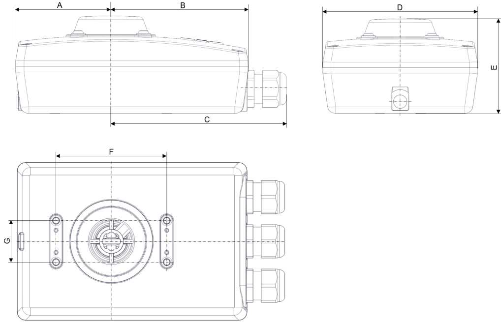
Şek. 4: Boyutlar
