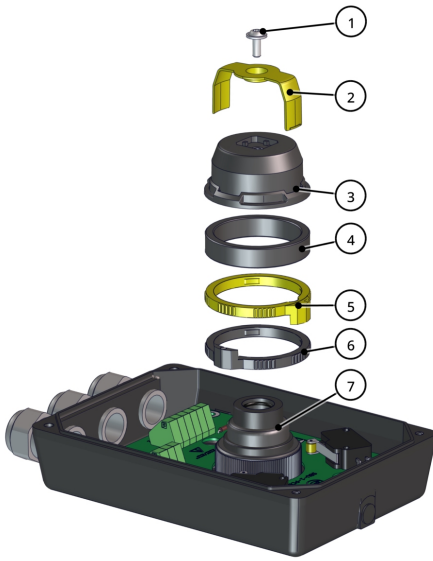
Şek. 8: Kam ayarı bileşenleri
