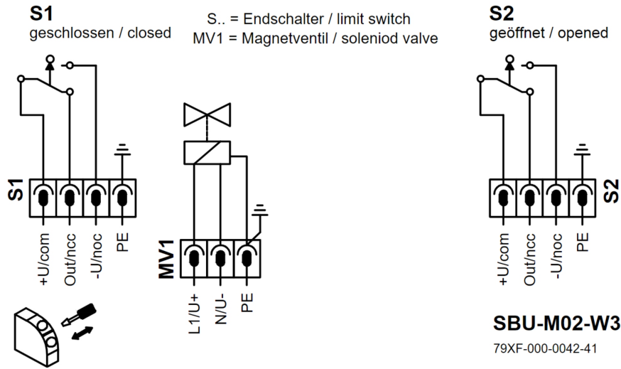
Şek. 7: SBU Basic elektrik şeması
