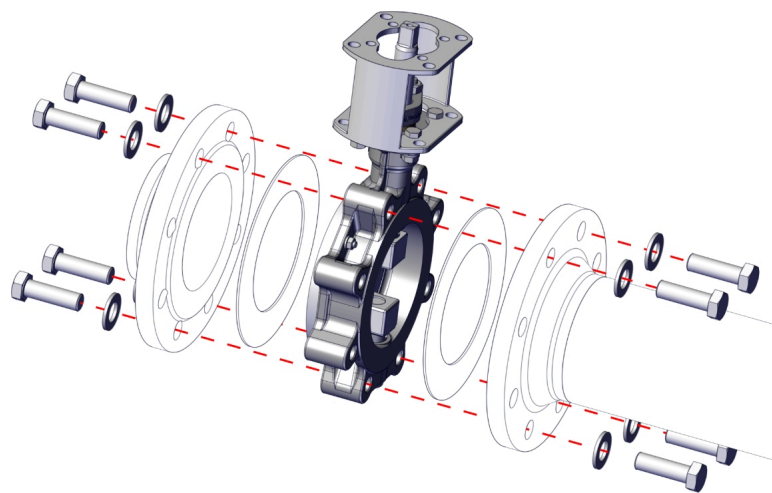
รูปที่ 8: การวางตำแหน่งวาล์วปีกผีเสื้อหน้าแปลนสวม
