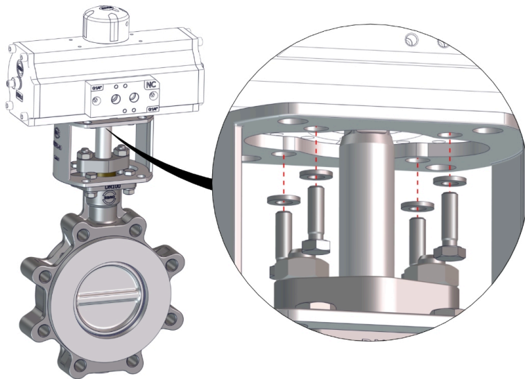
รูปที่ 7: หลักการประกอบชิ้นส่วน
