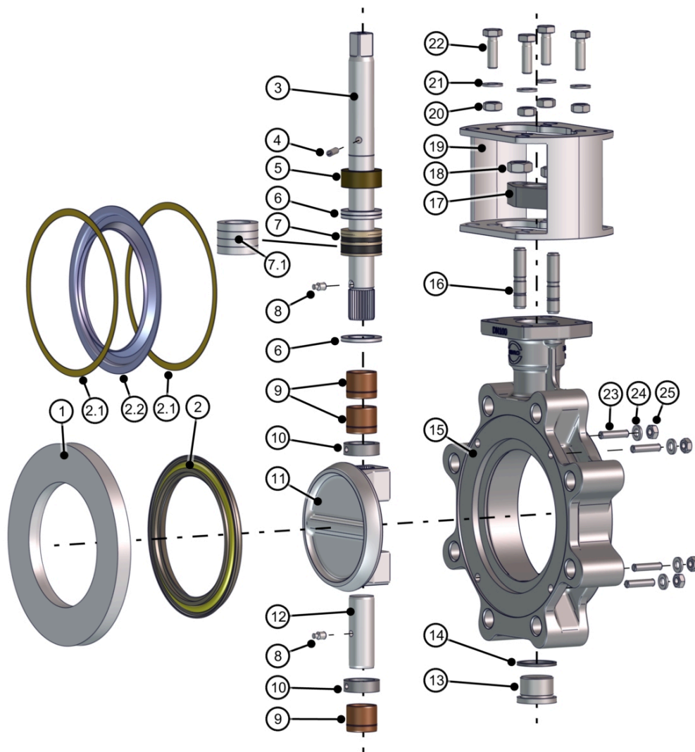
รูปที่ 15: รายการชิ้นส่วน HP114-HF
