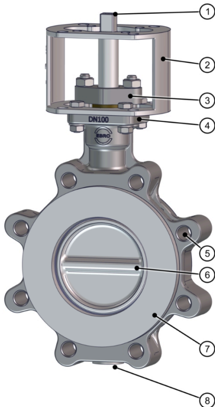
รูปที่ 2: ส่วนประกอบ
