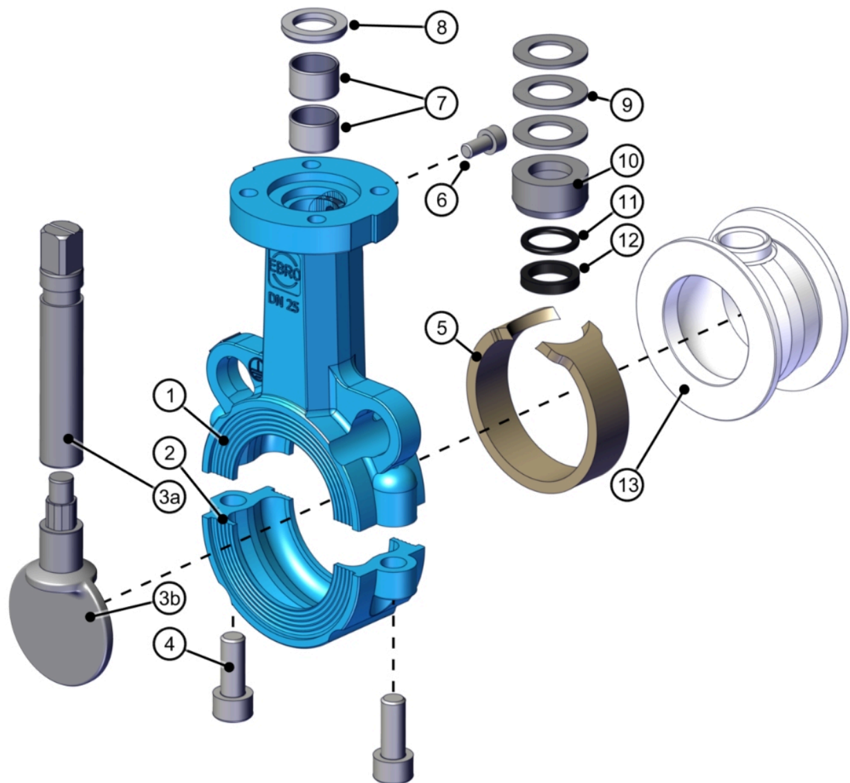
รูปที่ 15: รายการชิ้นส่วน T211-A ถึง DN32
