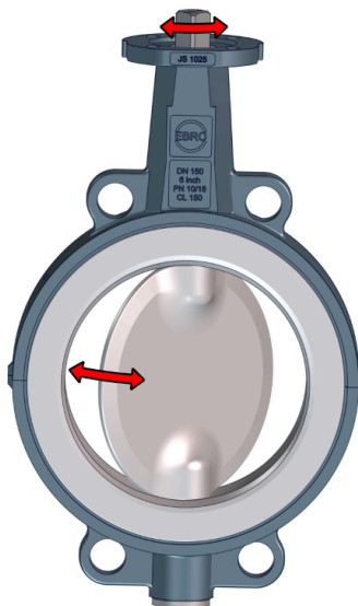
รูปที่ 4: ชิ้นส่วนที่เคลื่อนไหว
