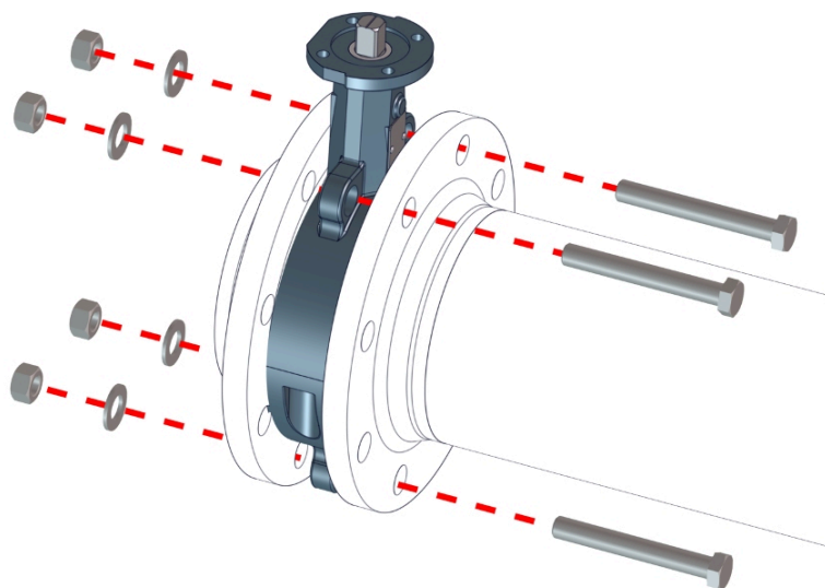
รูปที่ 8: Zwischenflanschklappe positionieren
