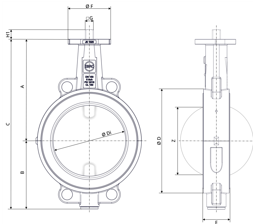
รูปที่ 3: ขนาดหลัก T211-A
