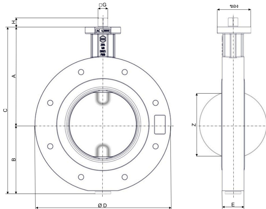
รูปที่ 3: ขนาดหลัก Z014-WN
