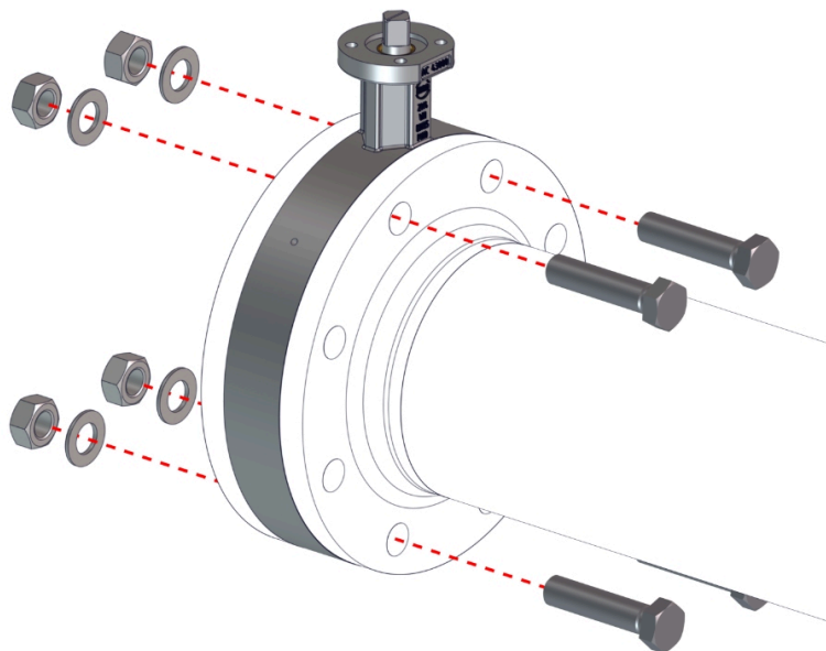
รูปที่ 8: การวางตำแหน่งแผ่นปิดหน้าแปลนแบบเดิม
