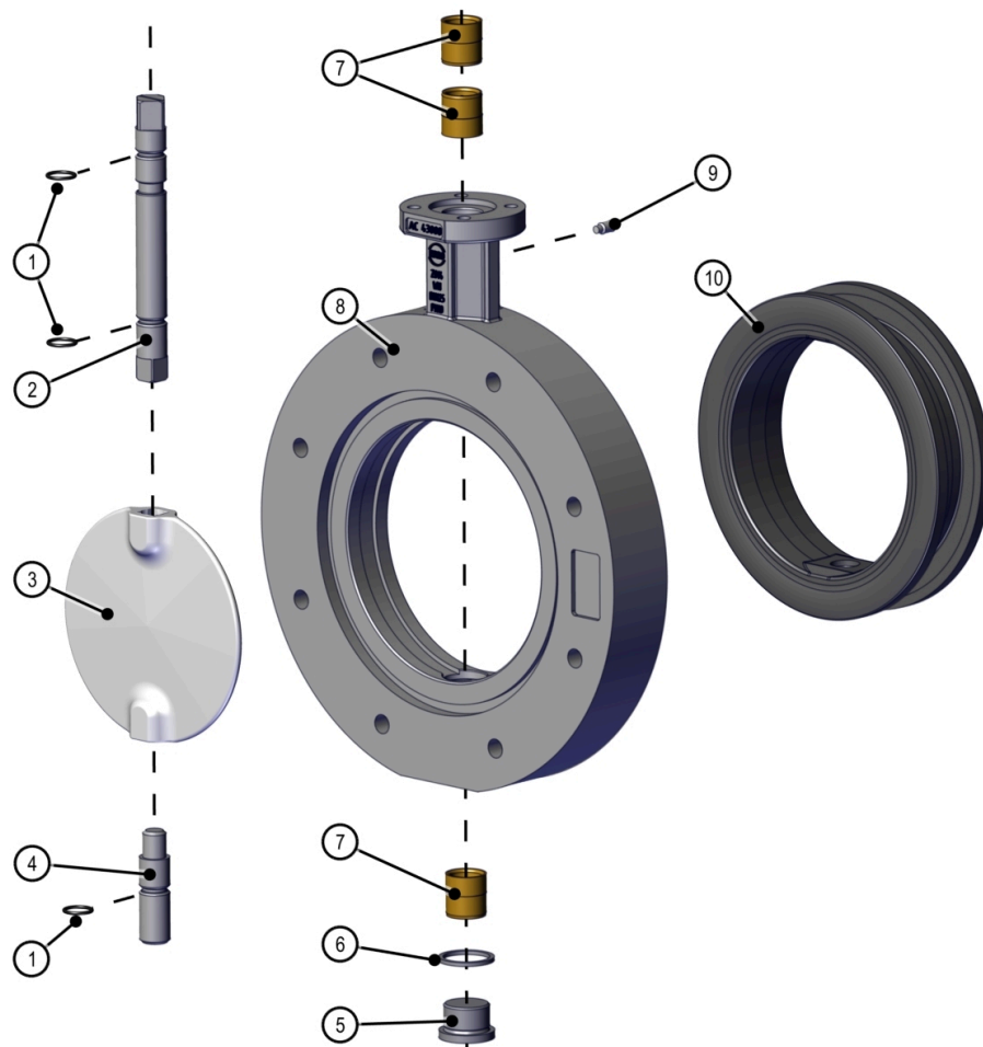
รูปที่ 15: รายการชิ้นส่วน Z014-WN
