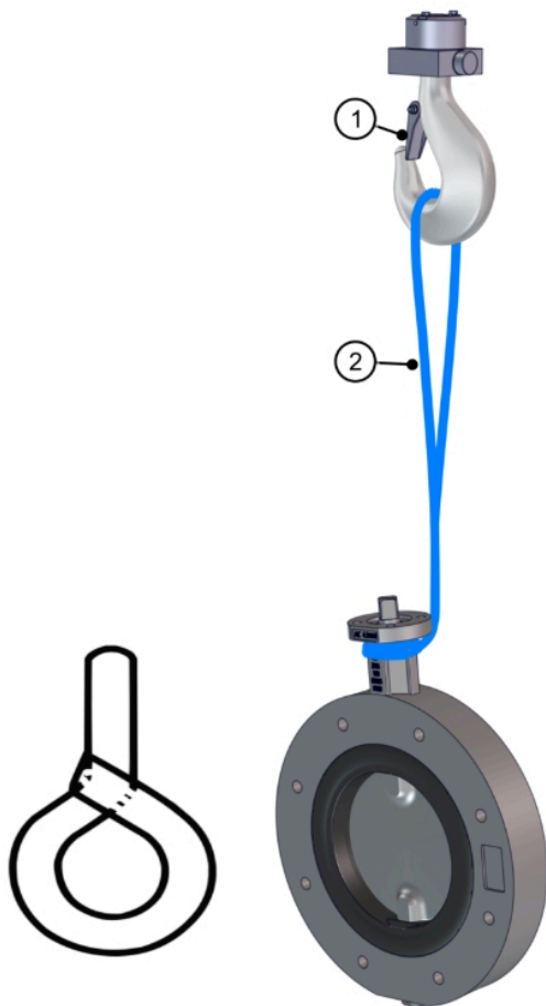
รูปที่ 6: การยกวาล์วปีกผีเสื้อหน้าแปลนเต็ม
