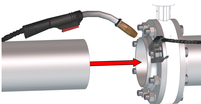
รูปที่ 10: เชื่อมท่อเข้ากับหน้าแปลน
