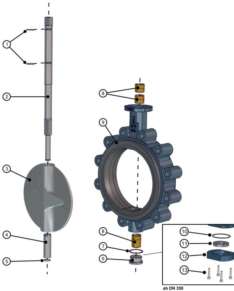
รูปที่ 16: รายการชิ้นส่วนเพลาทะลุ Z014-B TS
