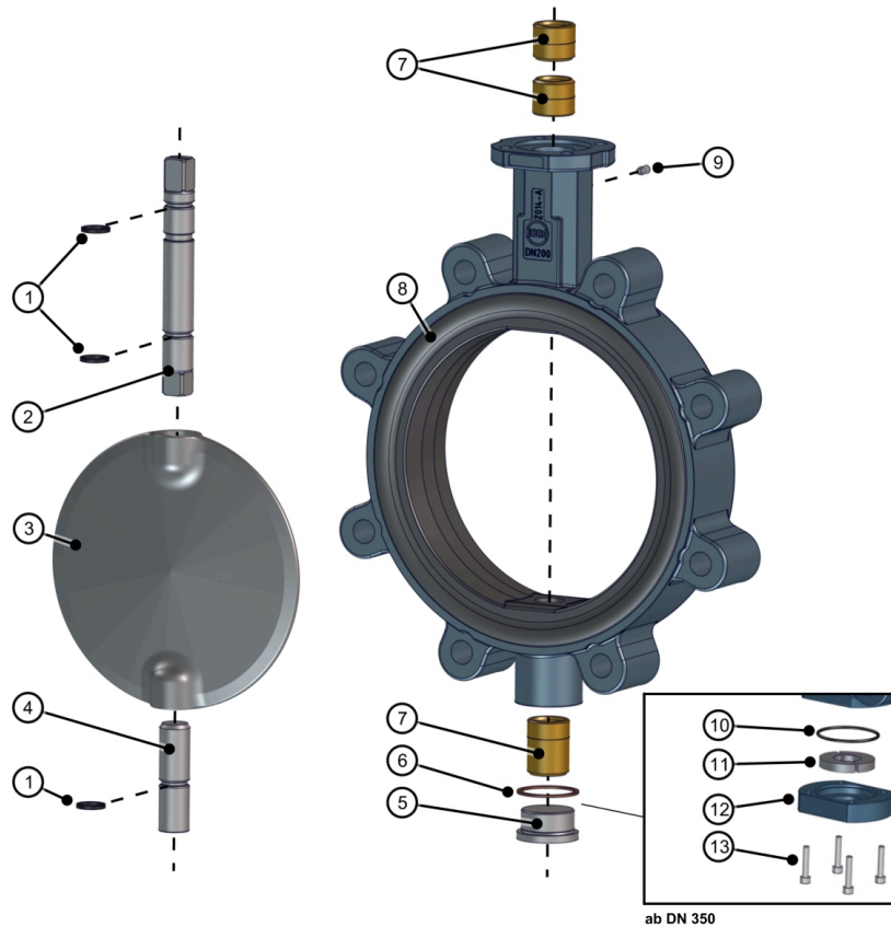
รูปที่ 15: รายการชิ้นส่วน Z014-B
