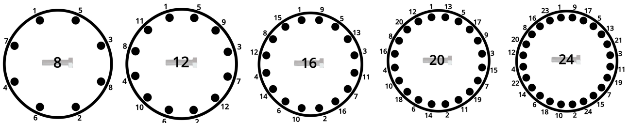
รูปที่ 12: ลำดับการติดตั้งหน้าแปลนท่อ
