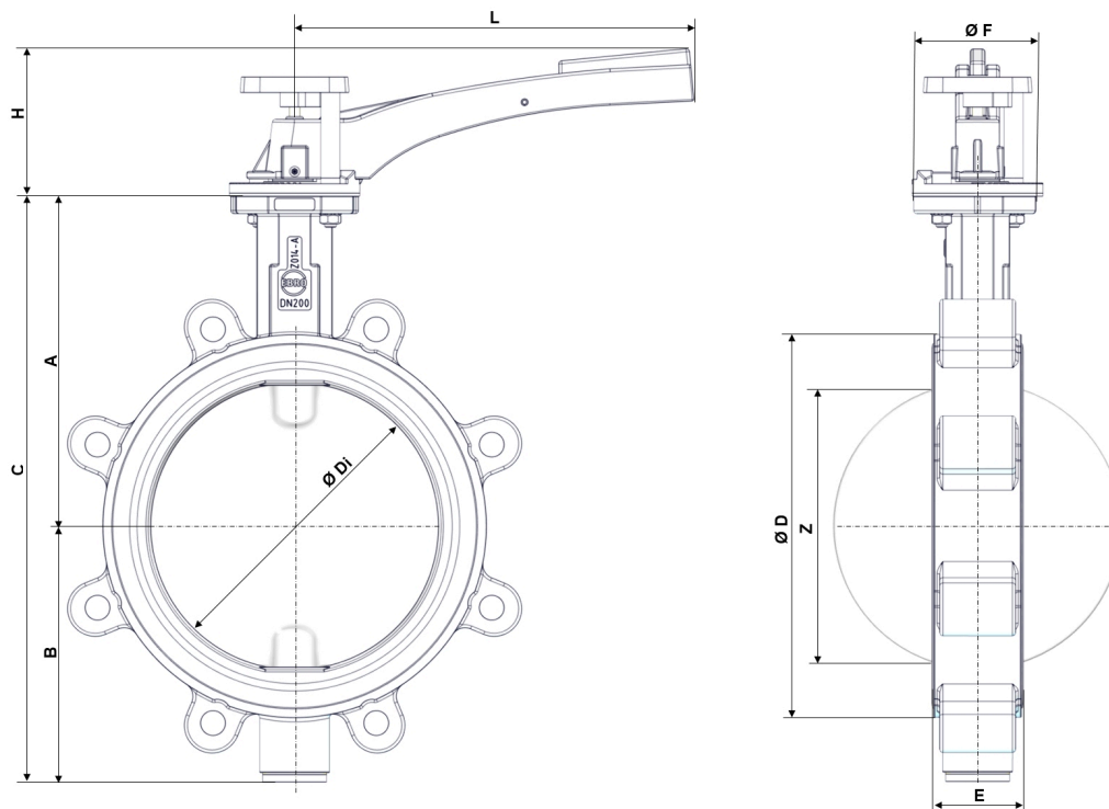
รูปที่ 3: ขนาดหลัก Z014-A THERM
