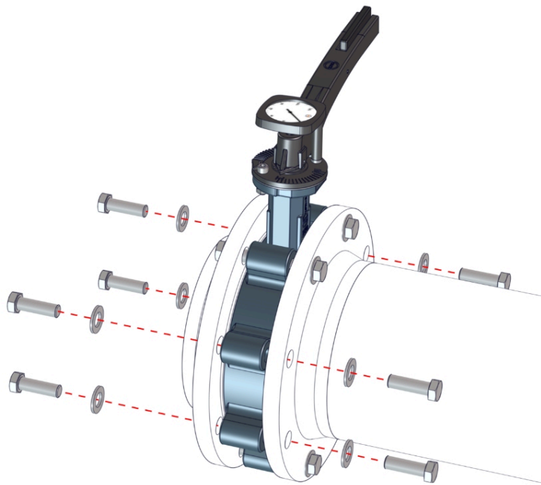
รูปที่ 9: ขั้นตอนการที่หน้าแปลน
