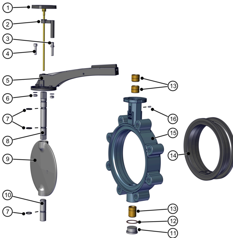
รูปที่ 16: รายการชิ้นส่วน Z014-A THERM
