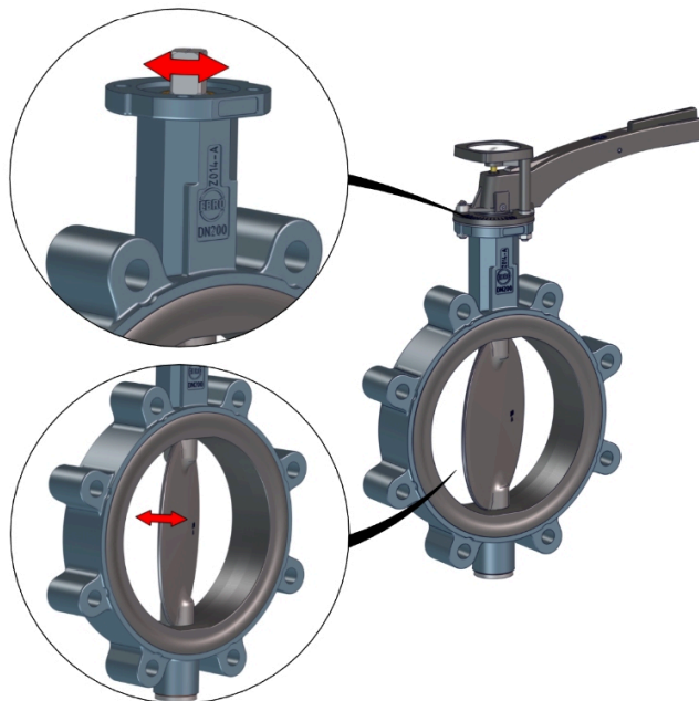
รูปที่ 4: ชิ้นส่วนที่เคลื่อนไหว
