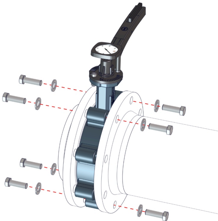
รูปที่ 8: การวางตำแหน่งวาล์วปีกผีเสื้อหน้าแปลนสวม
