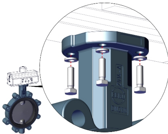
รูปที่ 7: หลักการประกอบชิ้นส่วน
