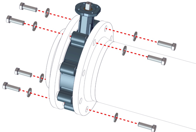
รูปที่ 8: การวางตำแหน่งวาล์วปีกผีเสื้อหน้าแปลนสวม
