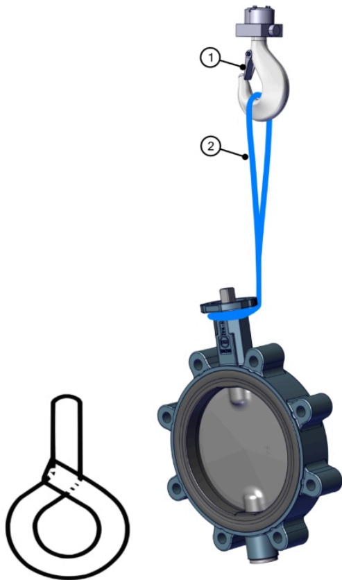
รูปที่ 6: การยกวาล์วปีกผีเสื้อหน้าแปลนสวม
