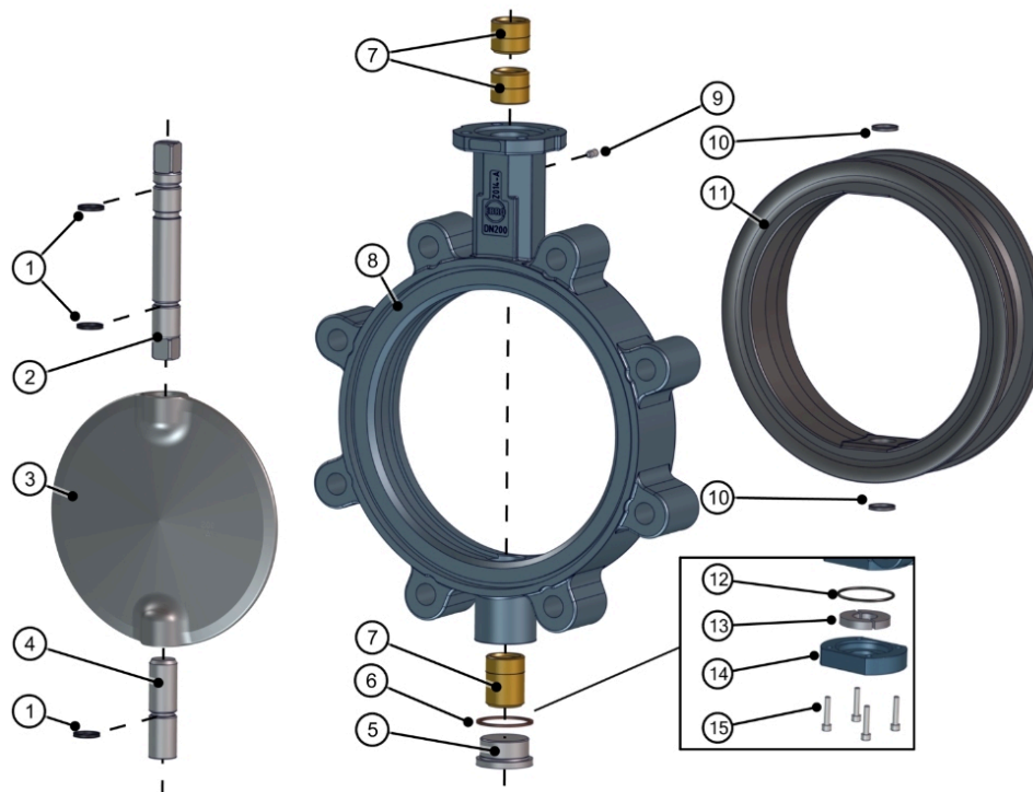
รูปที่ 15: รายการชิ้นส่วน Z014-A
