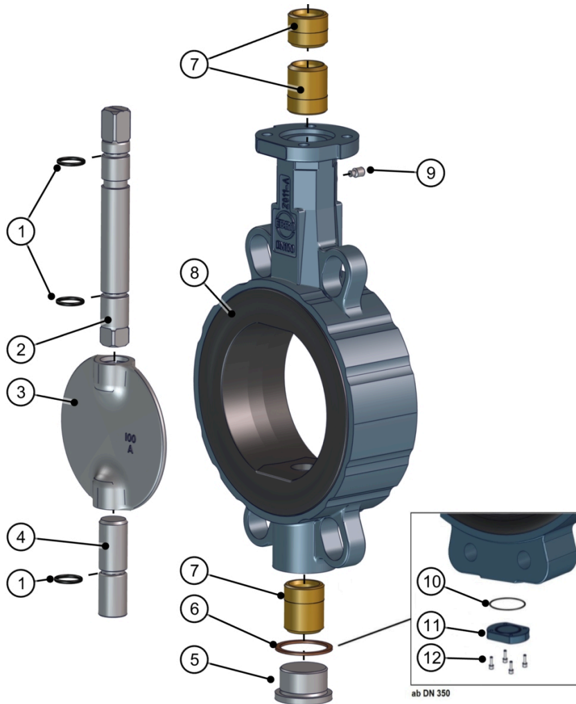
รูปที่ 15: รายการชิ้นส่วนเฟลาแยก Z011-B
