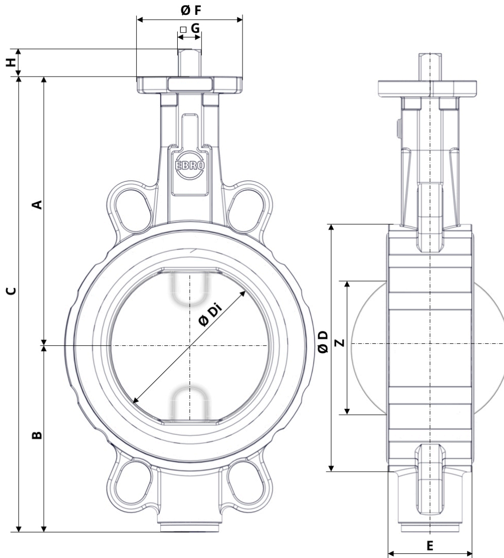
รูปที่ 3: ขนาดหลัก Z011-B
