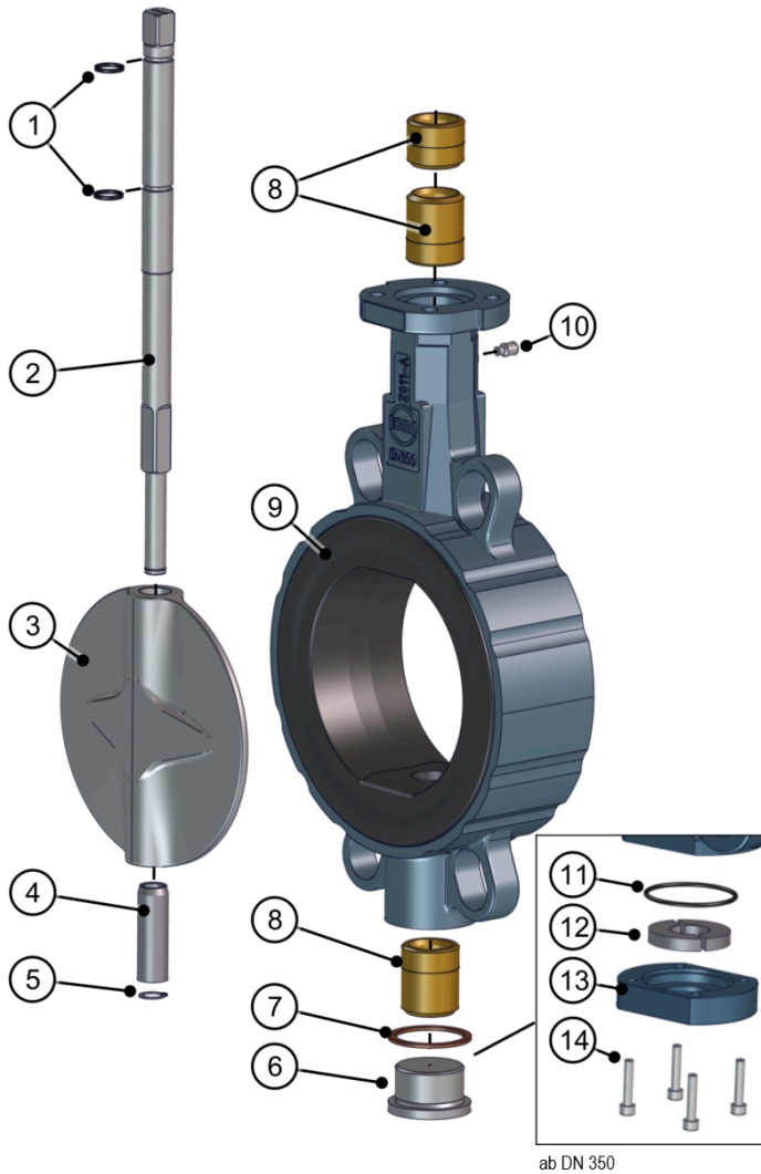
รูปที่ 16: รายการชิ้นส่วนเฟลา Z011-B TS
