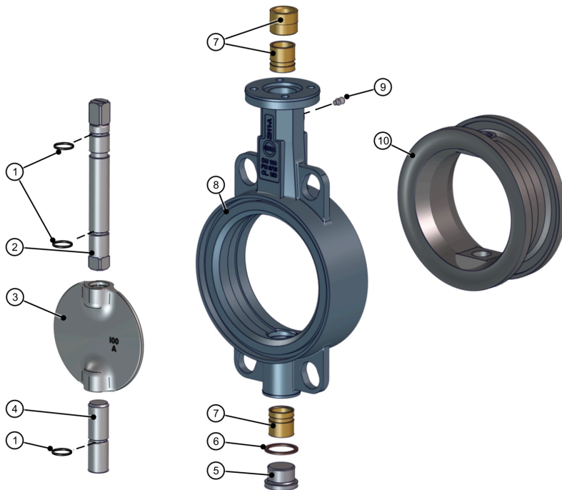
รูปที่ 15: รายการชิ้นส่วน Z011-AS
