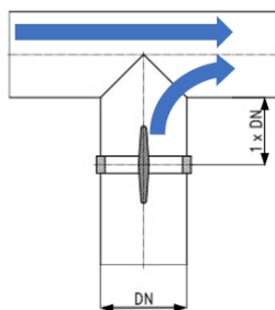
รูปที่ 11: ระยะทางถึงท่อแยก
