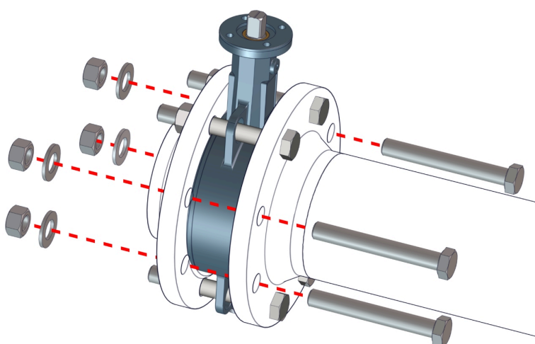
รูปที่ 9: ขันสกรูที่แผ่นหน้าแปลนกลาง
