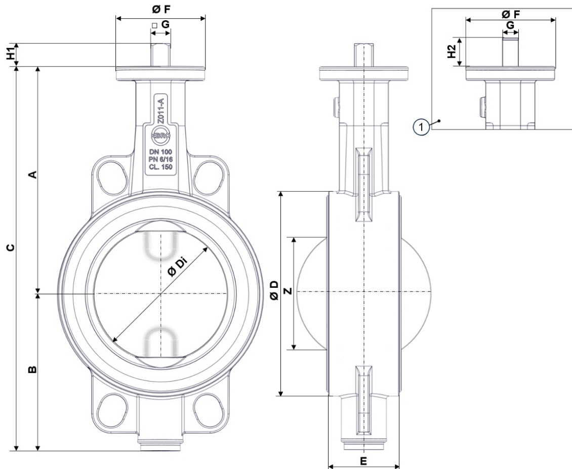
รูปที่ 3: ขนาดหลัก Z011-AS
