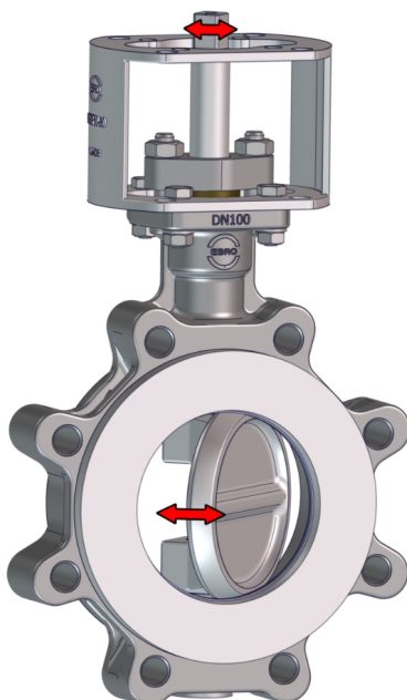
Fig. 4: Rörliga delar
