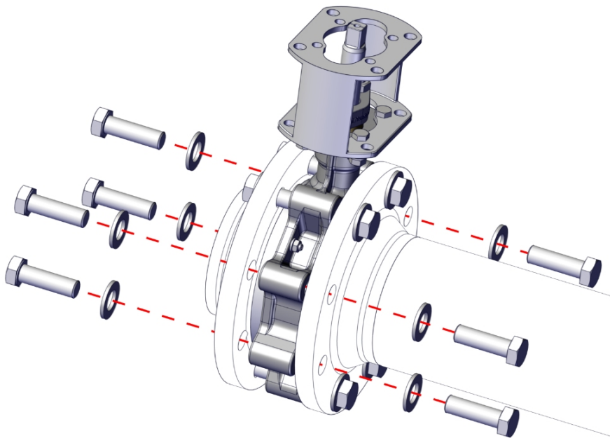
Fig. 9: Skruva fast spjällventil
