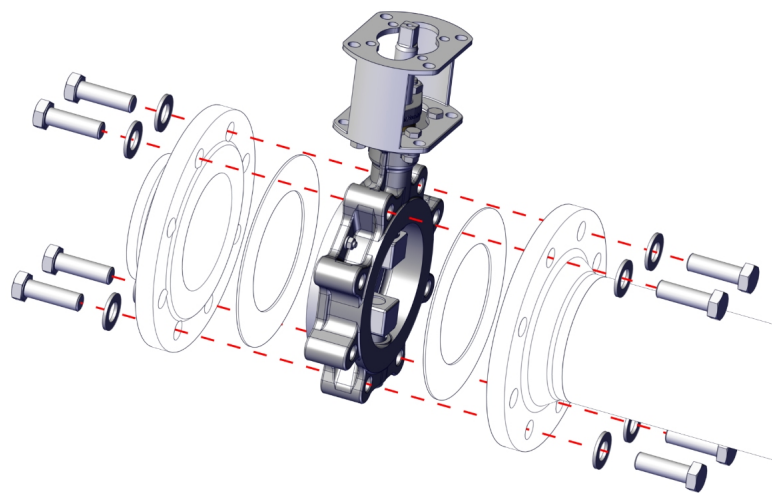
Fig. 8: Positionera spjällventil
