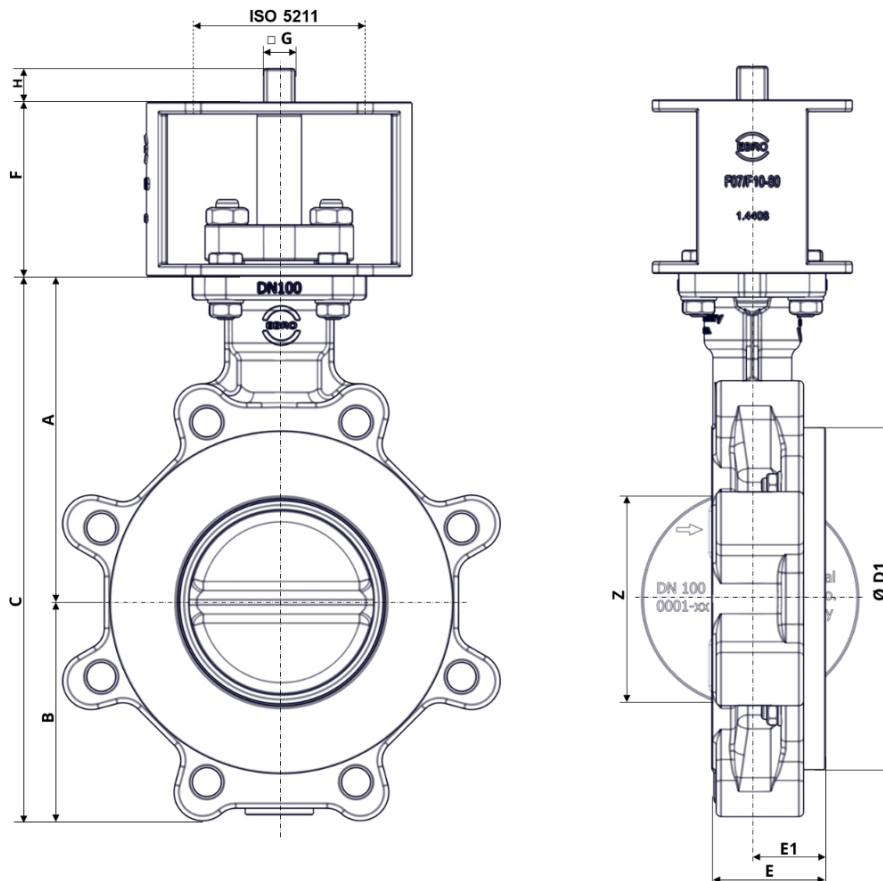
Fig. 3: Huvuddimensioner HP114-HF
