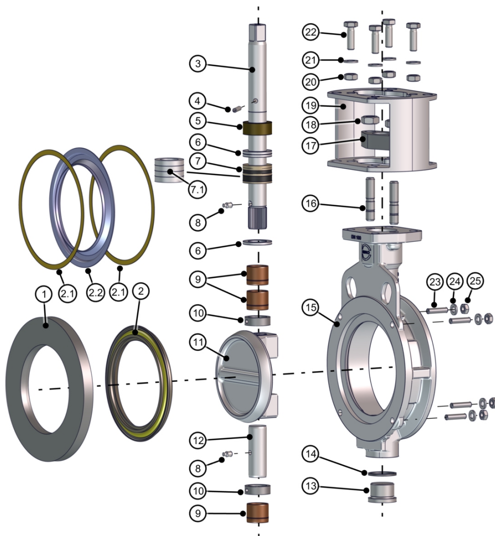
Fig. 15: Stycklista HP111-HF
