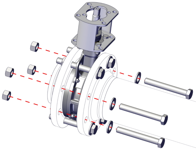
Fig. 9: Skruva fast mellanflänsspjäll
