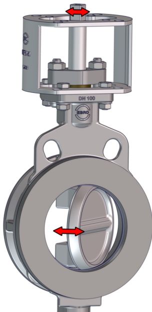
Fig. 4: Rörliga delar
