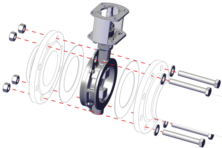
Fig. 8: Positionera mellanflänsspjäll
