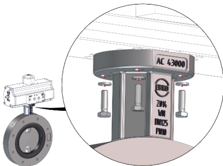
Fig. 7: Principillustration: montering av komponenter
