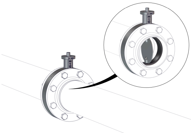
Fig. 13: Spola röret
