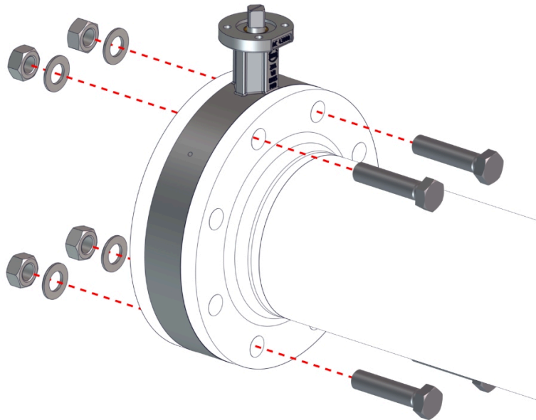
Fig. 8: Positionera spjällventil (fullflänsutförande)
