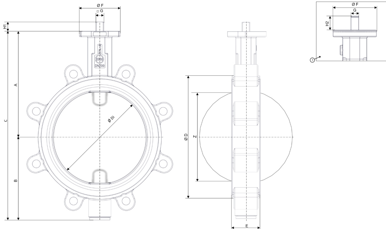
Fig. 3: Huvuddimensioner Z014-B
