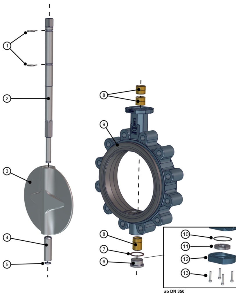
Fig. 16: Stycklista Z014-B TS-axel
