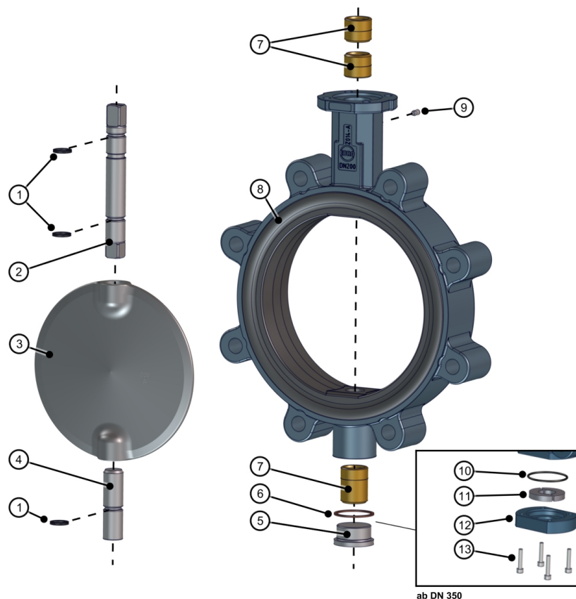
Fig. 15: Stycklista Z014-B
