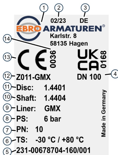
Fig. 1: exempel på märkskylt
