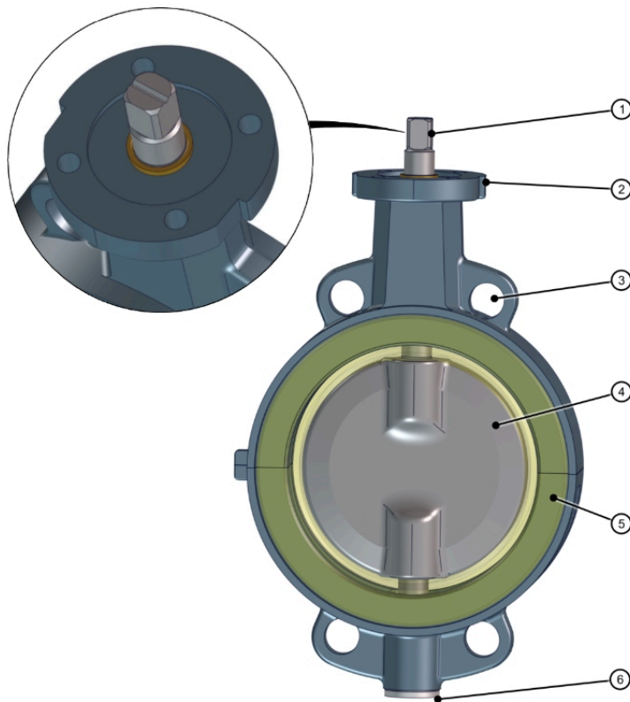
Fig. 2: Komponenter
