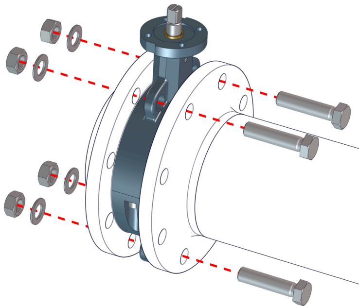
Fig. 8: Positionera mellanflänsspjäll
