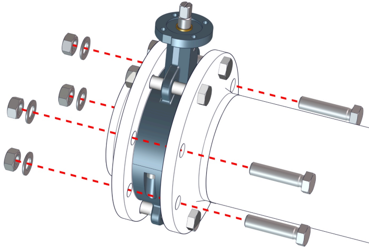
Fig. 9: Skruva fast mellanflänsspjäll
