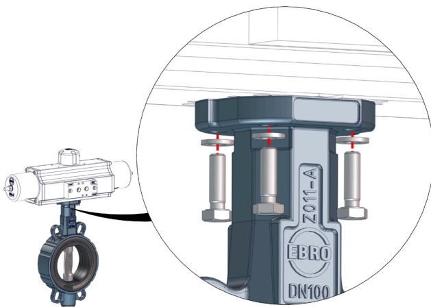
Fig. 7: Principillustration: montering av komponenter
