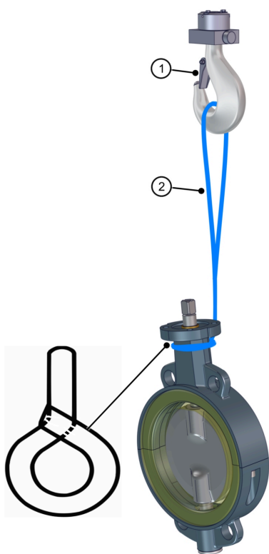
Fig. 6: Kranlyft av mellanflänsspjäll
