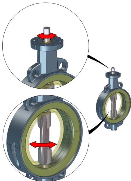
Fig. 4: Rörliga delar
