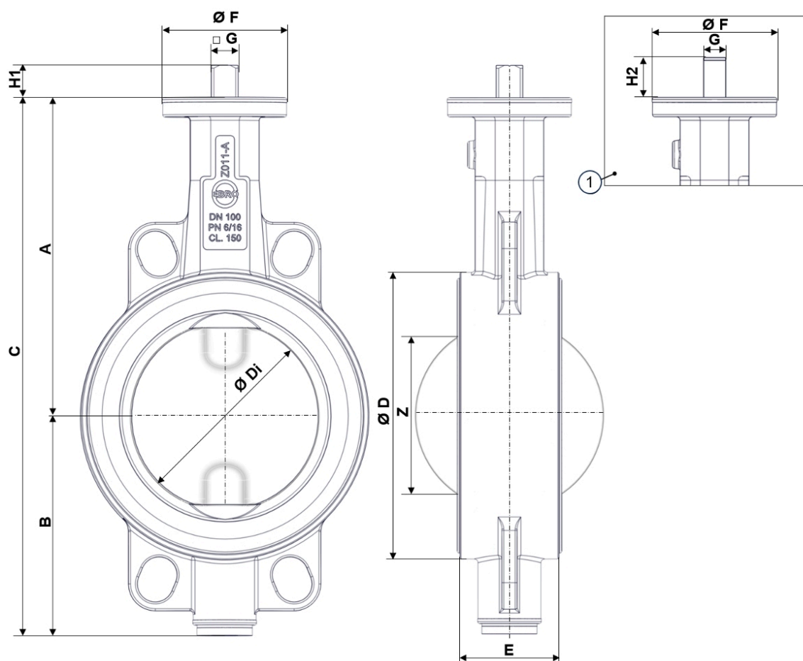
Fig. 3: Huvuddimensioner Z011-AS
