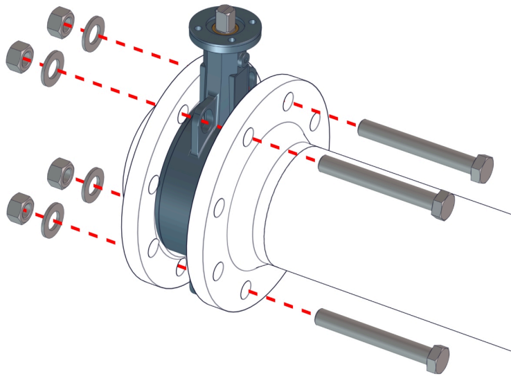
Fig. 8: Positionera mellanflänsspjäll
