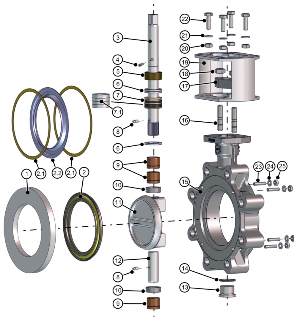
Fig. 15: Lista de piezas HP114-HF
