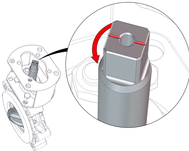
Fig. 14: Dirección de accionamiento
