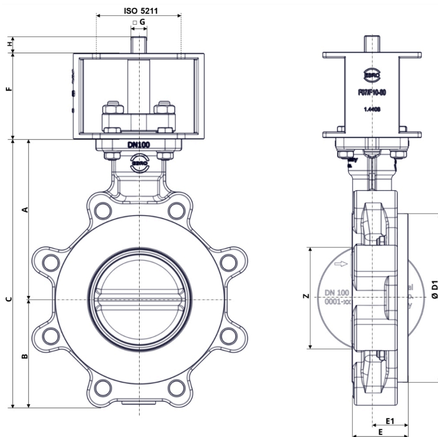
Fig. 3: Dimensiones principales HP114-HF
