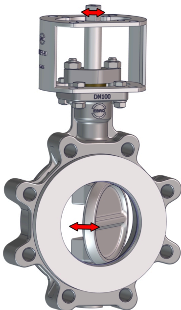
Fig. 4: Piezas móviles
