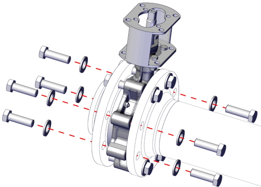
Fig. 9: Atornillar válvula de mariposa tipo lug
