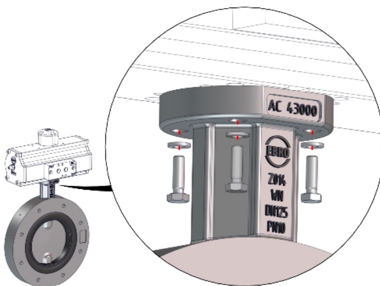
Fig. 7: Principio de montaje de componentes
