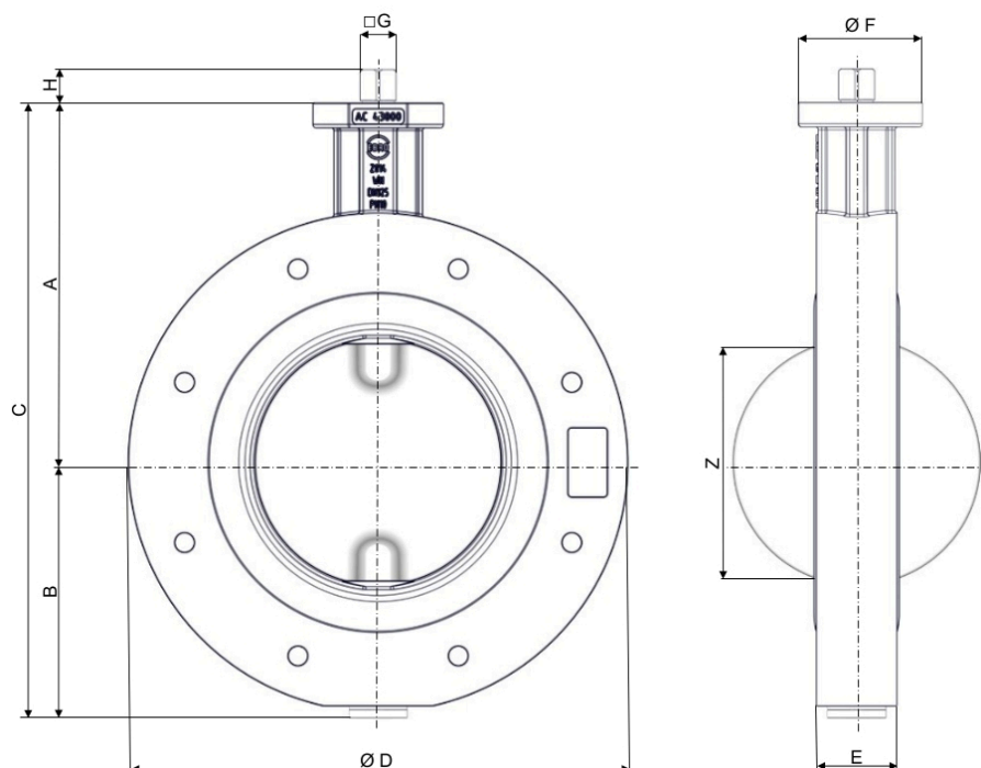
Fig. 3: Dimensiones principales Z014-WN
