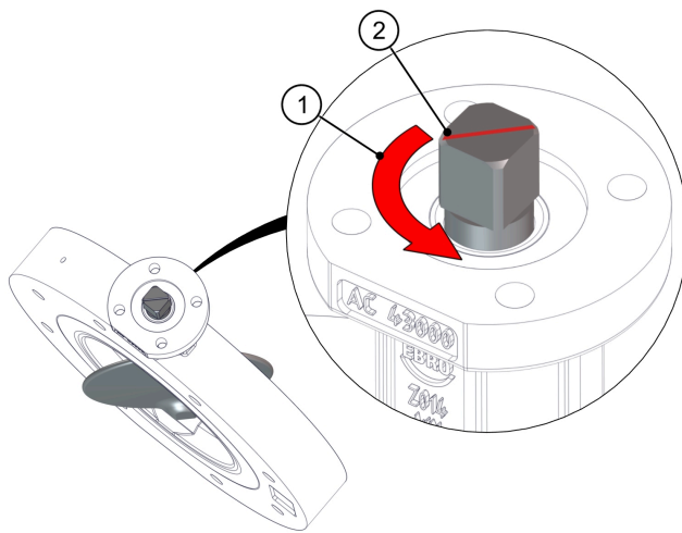
Fig. 14: Dirección de accionamiento
