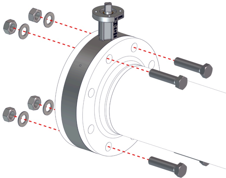
Fig. 8: Posicionar válvula de brida completa
