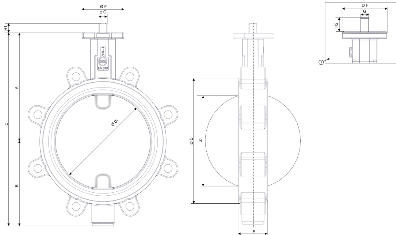
Fig. 3: Dimensiones principales Z014-B
