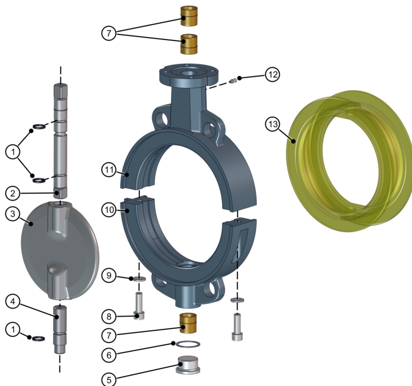
Fig. 15: Lista de piezas Z011-GMX
