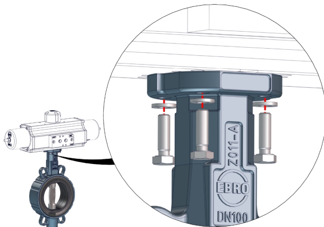
Fig. 7: Principio de montaje de componentes
