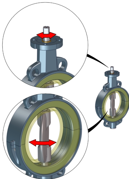
Fig. 4: Piezas móviles
