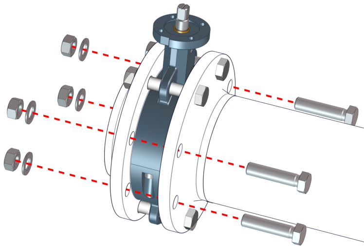
Fig. 9: Atornillar la válvula de mariposa tipo wafer
