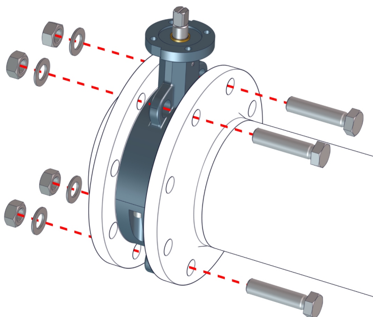
Fig. 8: Posicionar la válvula de mariposa tipo wafer
