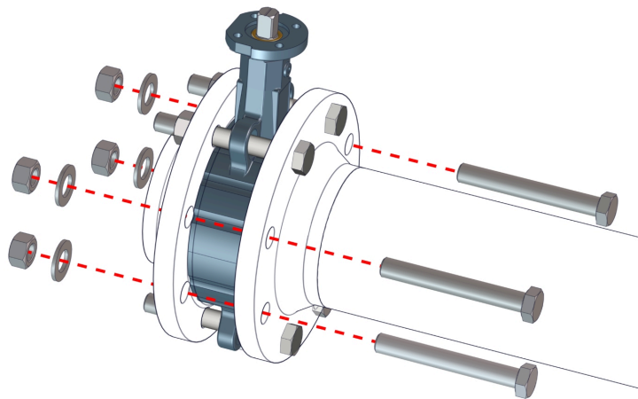
Fig. 9: Atornillar la válvula de mariposa tipo wafer
