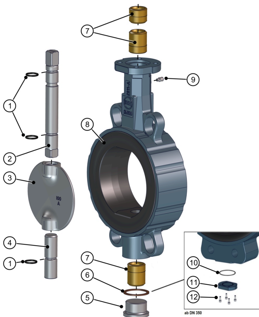
Fig. 15: Lista de piezas Z011-B eje dividido
