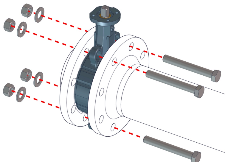
Fig. 8: Posicionar la válvula de mariposa tipo wafer
