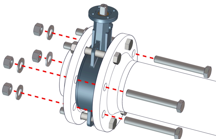
Fig. 9: Atornillar la válvula de mariposa tipo wafer
