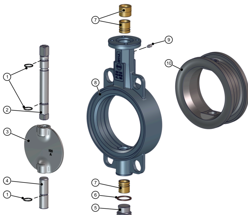
Fig. 15: Lista de piezas Z011-AS
