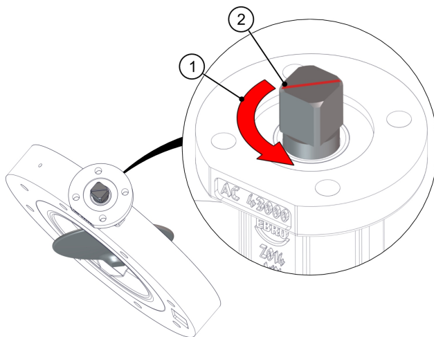
Sl. 14: Smer aktiviranja
