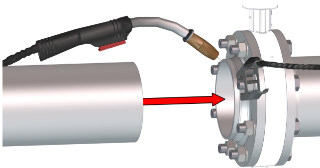
Sl. 10: Varenje cevi s prirobnico
