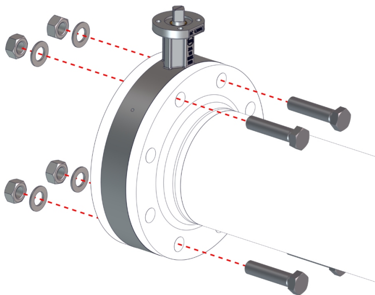
Sl. 8: Pozicioniranje lopute s polno prirobnico
