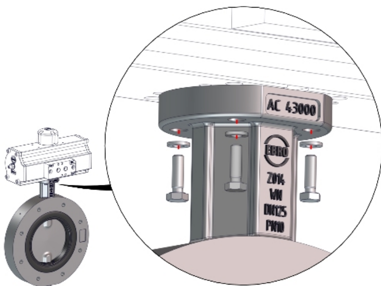
Sl. 7: Načelo montaže komponent
