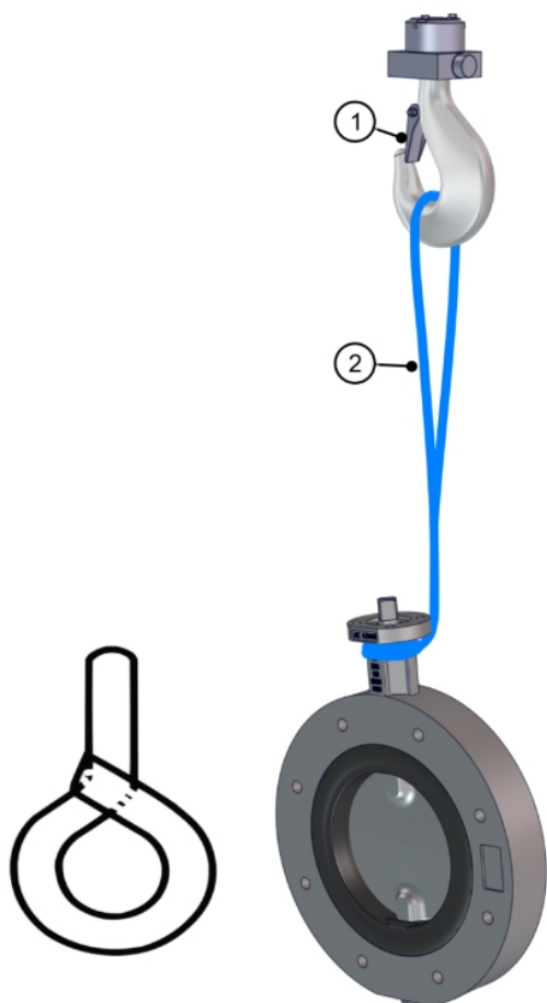
Sl. 6: Dvig lopute s polno prirobnico z žerjavom
