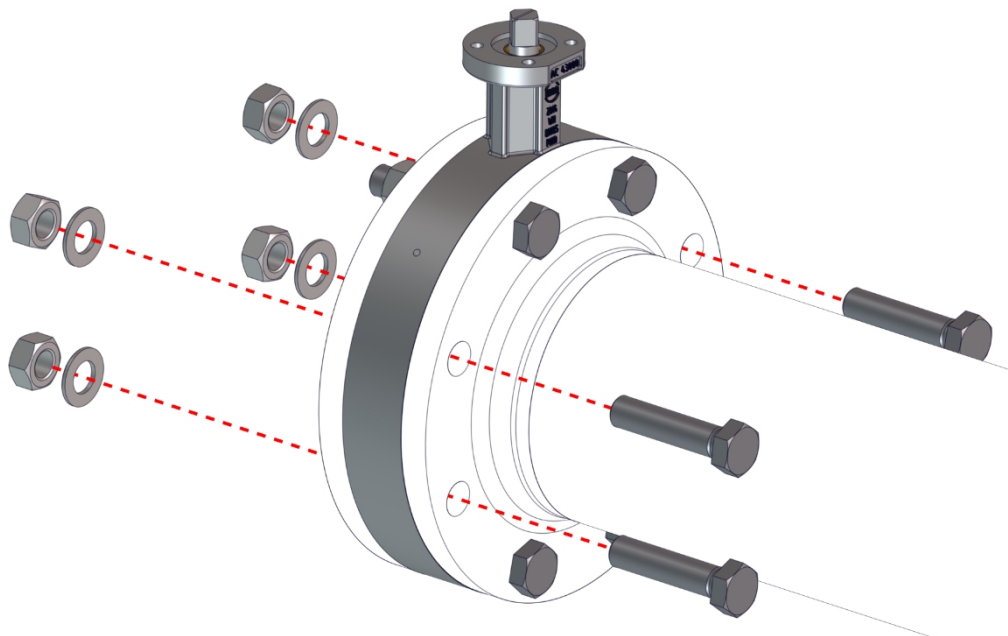
Sl. 9: Privijanje lopute s polno prirobnico
