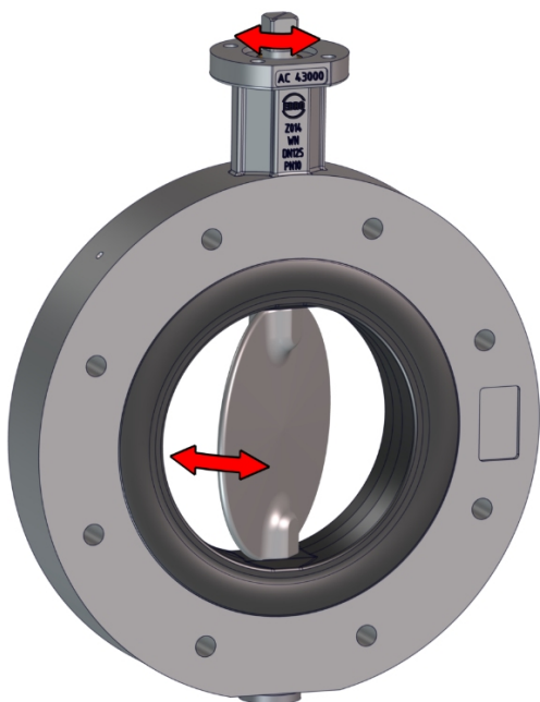
Sl. 4: Premični deli
