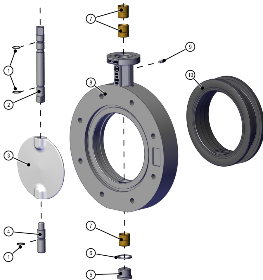
Sl. 15: Kosovni seznam Z014-WN
