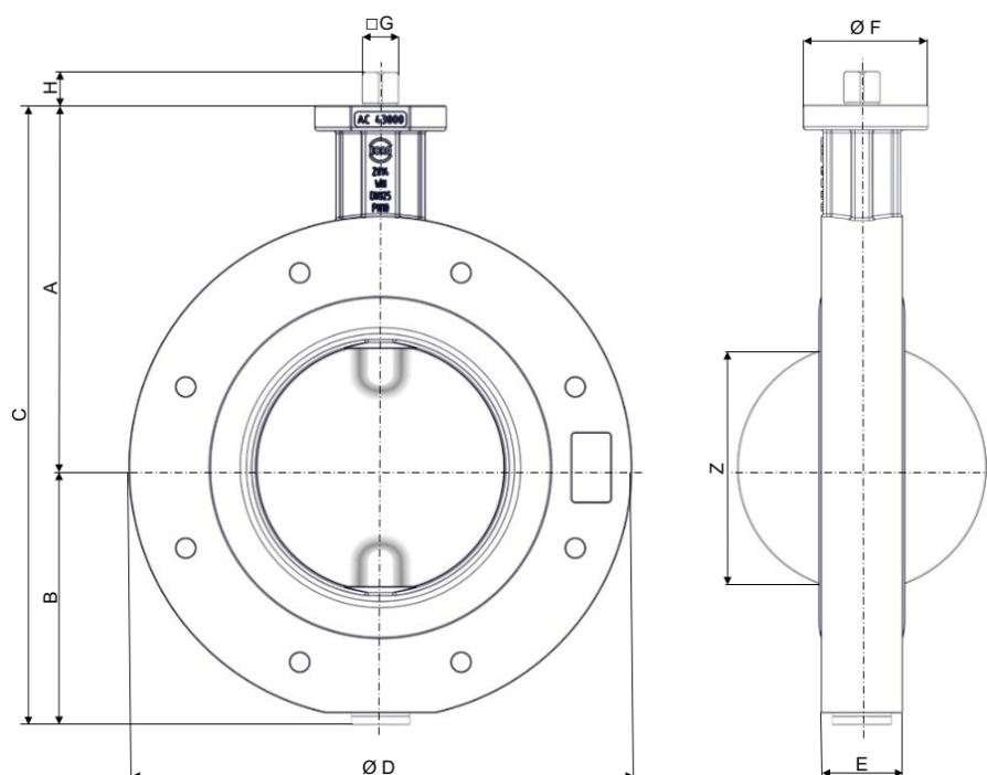
Sl. 3: Glavne dimenzije Z014-WN
