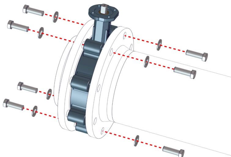
Sl. 8: Pozicioniranje lopute z naležno prirobnico
