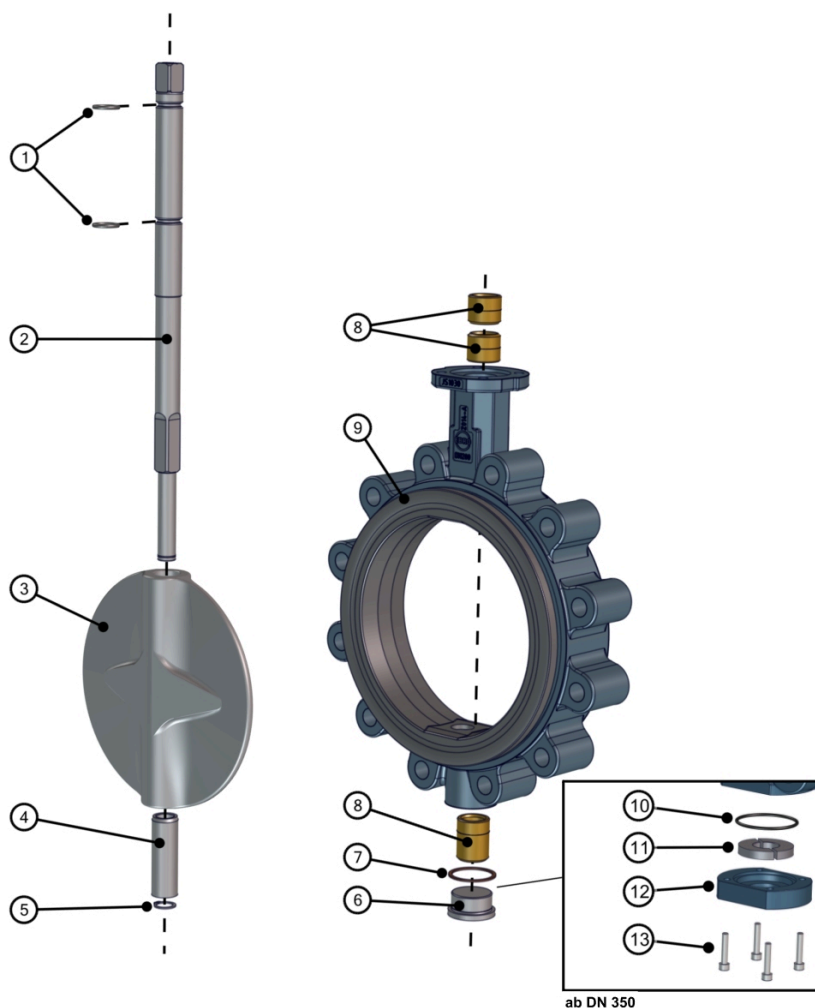
Sl. 16: Kosovni seznam Z014-B TS-gred
