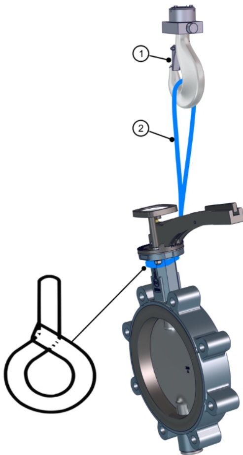
Sl. 6: Dvig lopute s prirobnico z žerjavom
