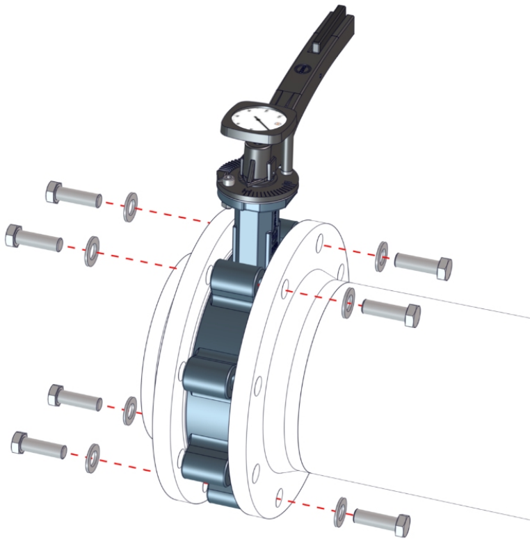
Sl. 8: Pozicioniranje lopute z naležno prirobnico
