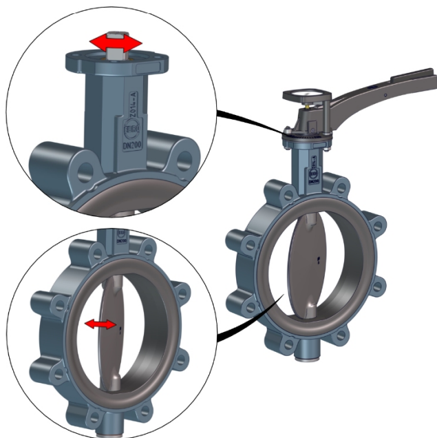
Sl. 4: Premični deli
