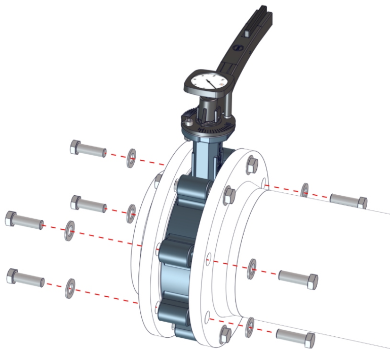
Sl. 9: Privijanje lopute z naležno prirobnico
