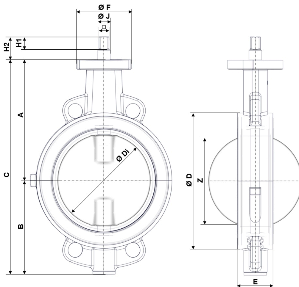
Sl. 3: Glavne dimenzije Z011-GMX
