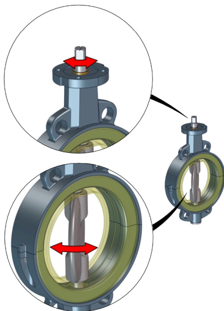
Sl. 4: Premični deli
