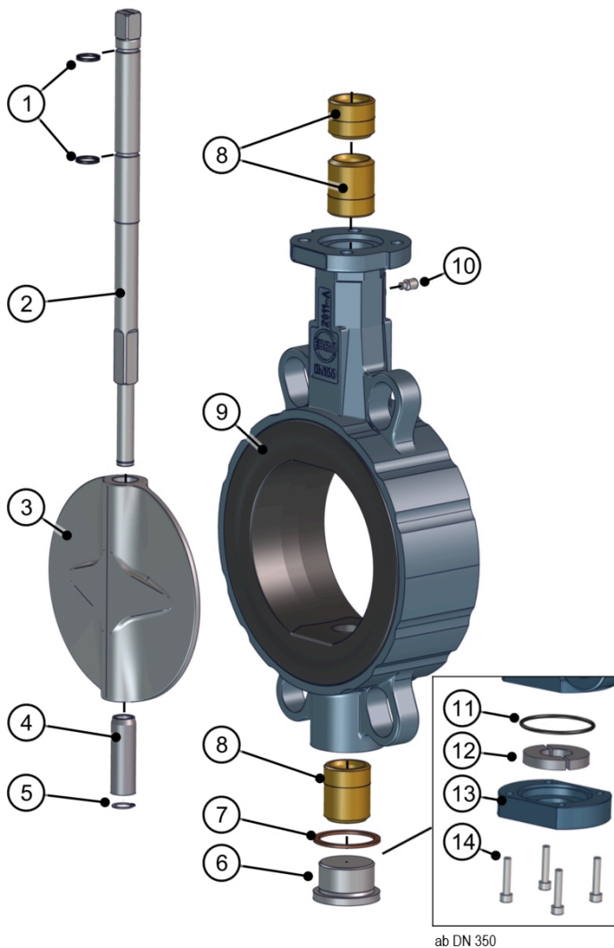
Sl. 16: Kosovni seznam Z011-B TS-gred
