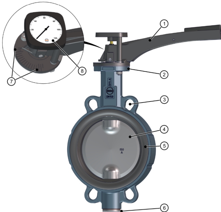
Sl. 2: Komponente
