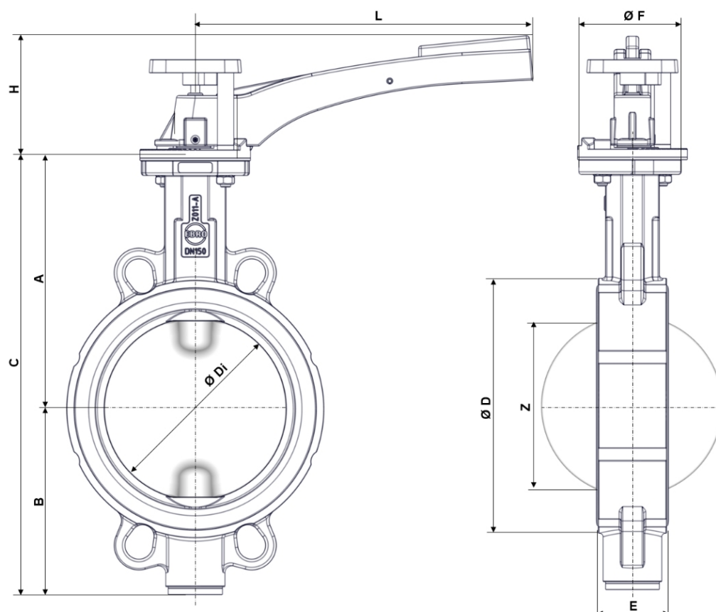
Sl. 3: Glavne dimenzije Z011-A THERM
