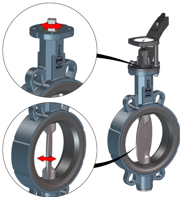
Sl. 4: Premični deli
