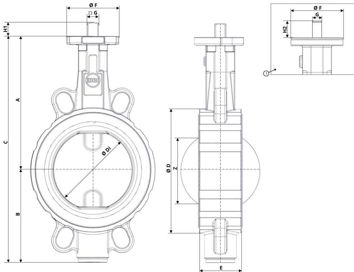
Sl. 3: Glavne dimenzije Z011-A
