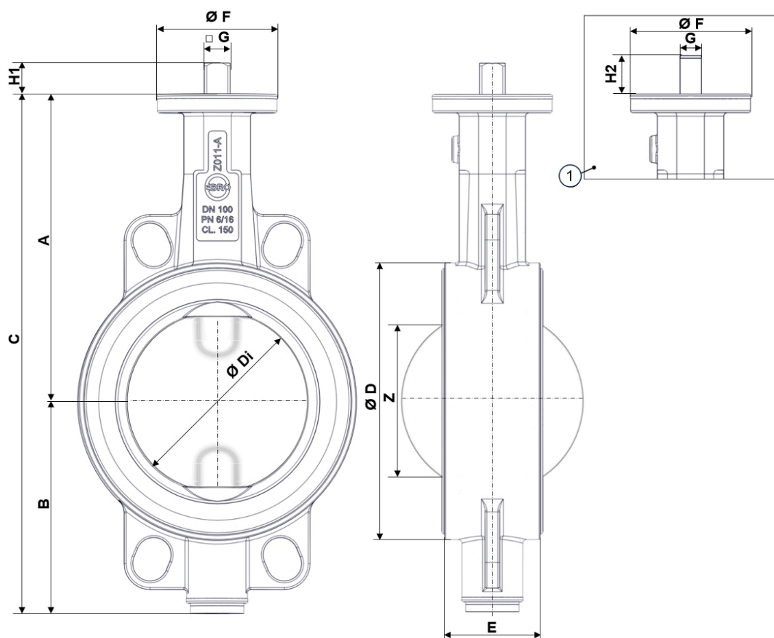
Sl. 3: Glavne dimenzije Z011-AS
