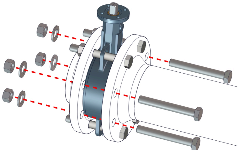
Sl. 9: Privijanje lopute z vmesno prirobnico
