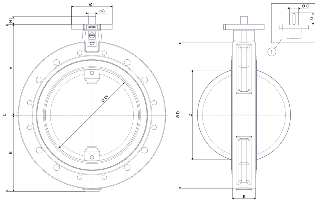
Obr. 3: Hlavné rozmery T212-A
