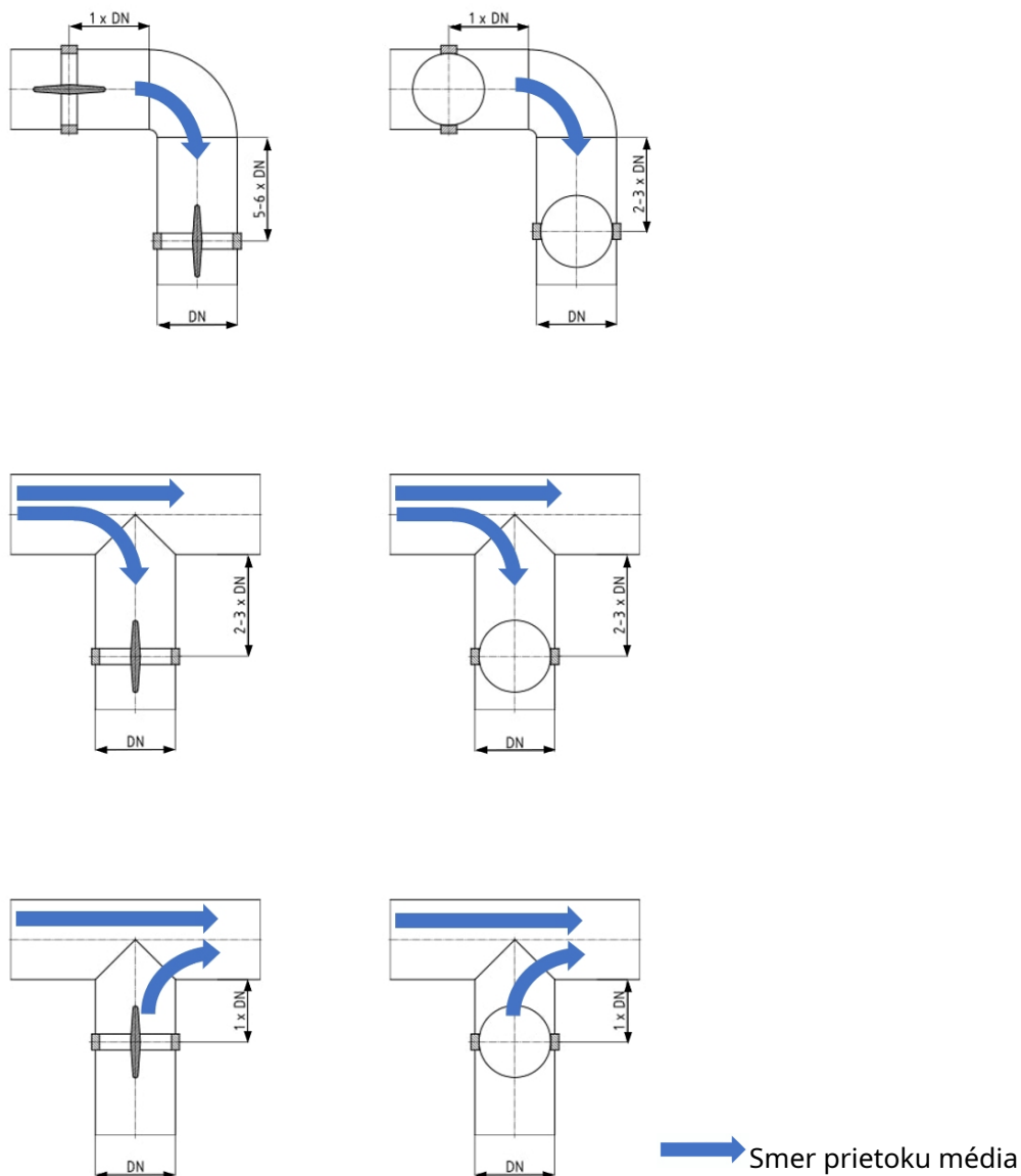
Obr. 11: Vzdialenosti k odbočkám potrubia
