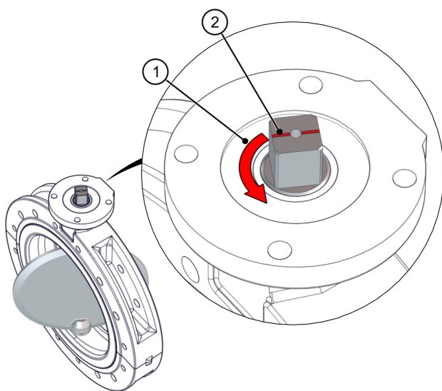
Obr. 14: Smer ovládania
