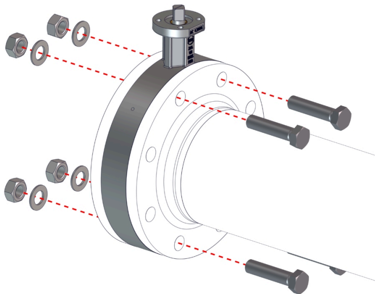
Obr. 8: Umiestnenie klapky s plnou prírubou
