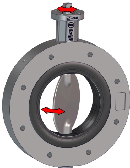
Obr. 4: Pohyblivé časti
