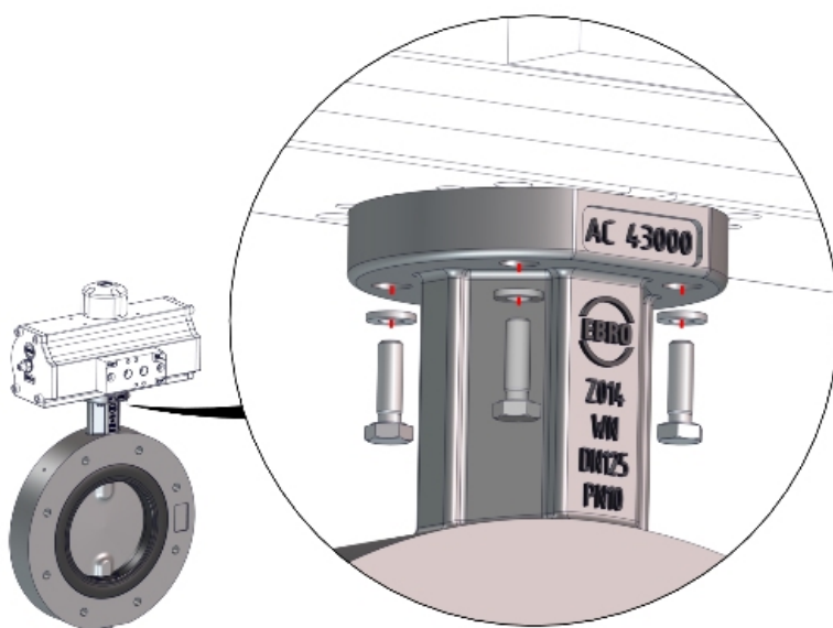
Obr. 7: Princíp ako montovať komponenty
