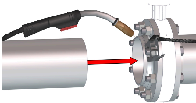
Obr. 10: Zváranie potrubia s prírubou
