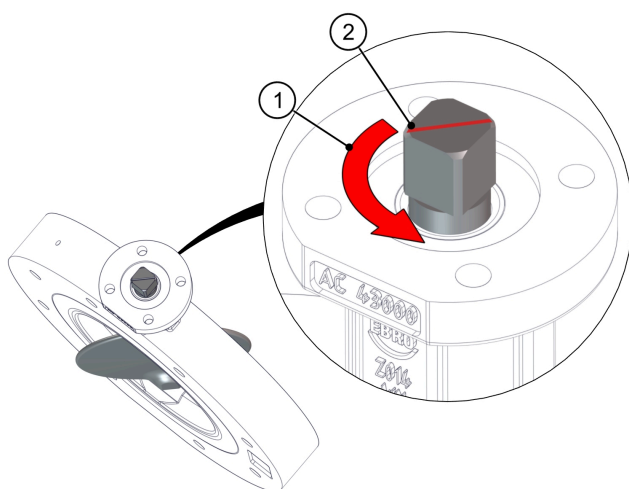
Obr. 14: Smer ovládania
