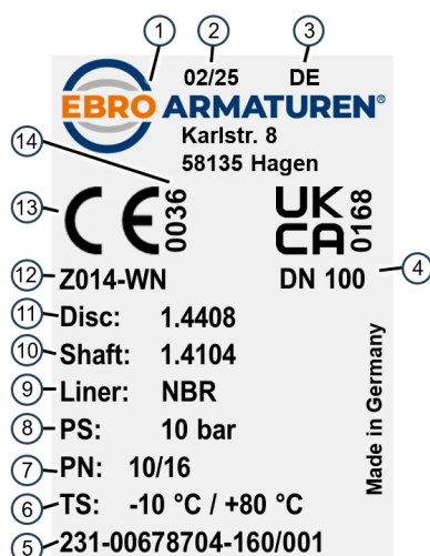
Obr. 1: Príklad typového štítku
