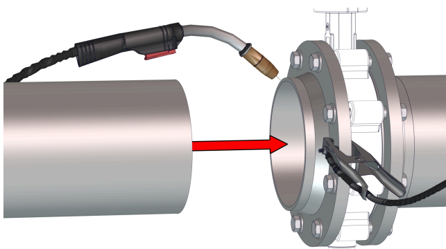
Obr. 10: Zváranie potrubia s prírubou
