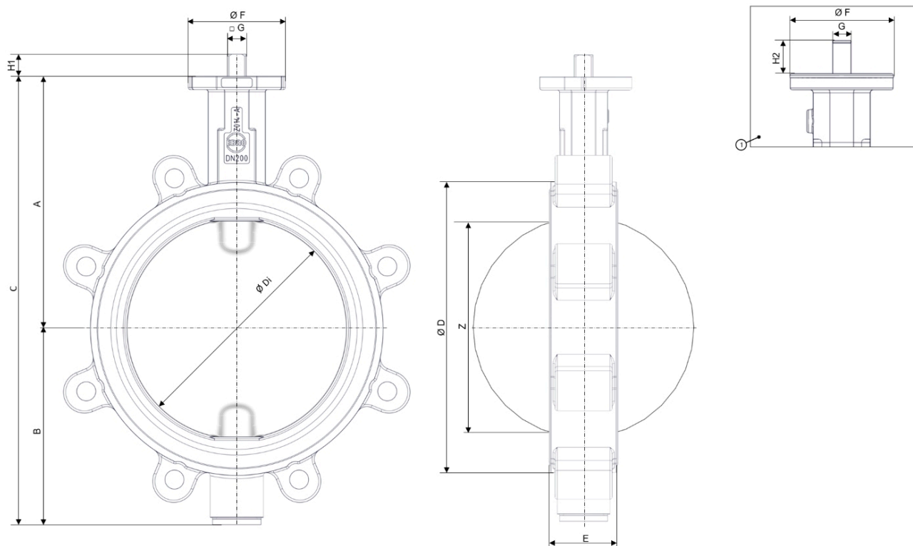
Obr. 3: Hlavné rozmery Z014-B
