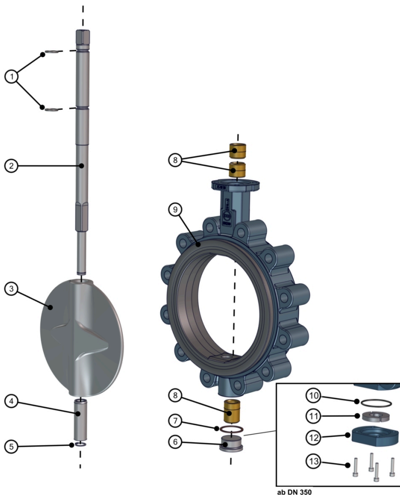
Obr. 16: Kusovník, Z014-B hriadeľ TS
