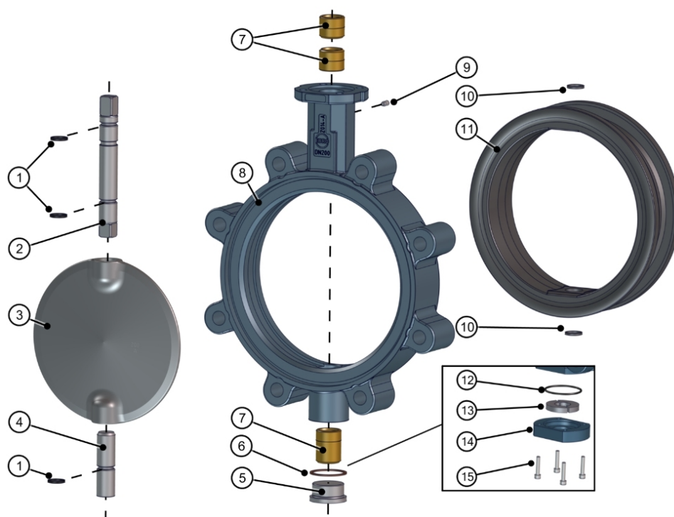
Obr. 15: Kusovník Z014-A
