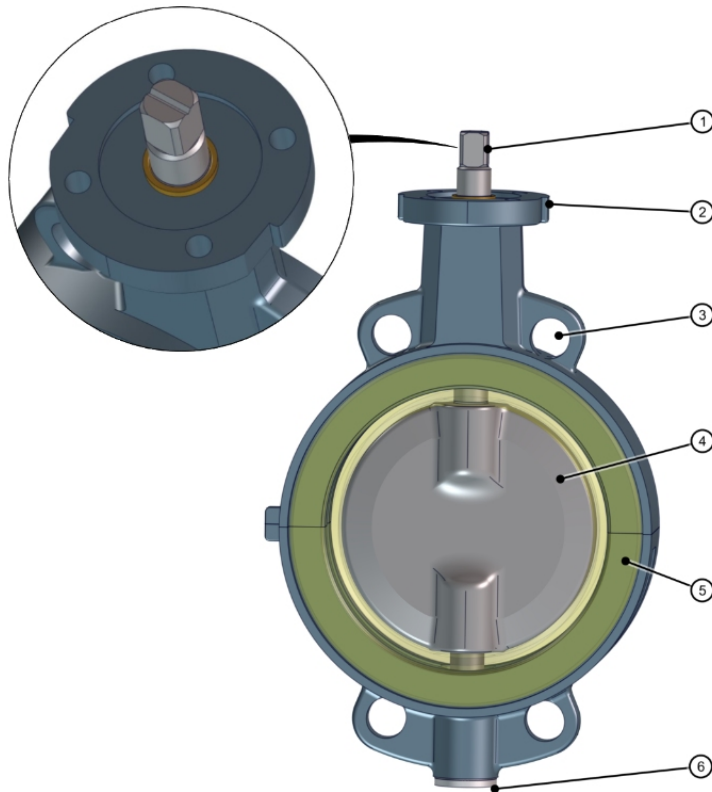
Obr. 2: Komponenty
