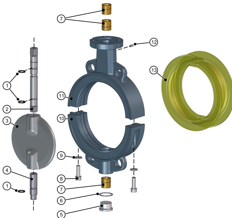
Obr. 15: Kusovník Z011-GMX
