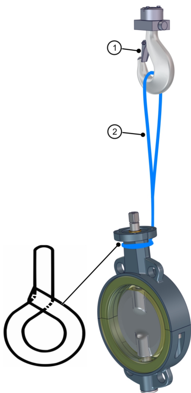
Obr. 6: Preprava medziprírubovej klapky žeriavom
