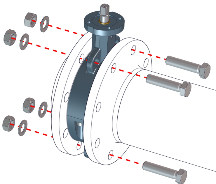
Obr. 8: Umiestnenie medziprírubovej klapky
