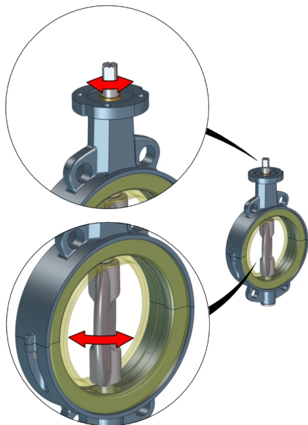
Obr. 4: Pohyblivé časti
