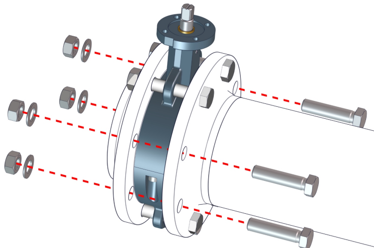
Obr. 9: Skrutkovanie medziprírubovej klapky
