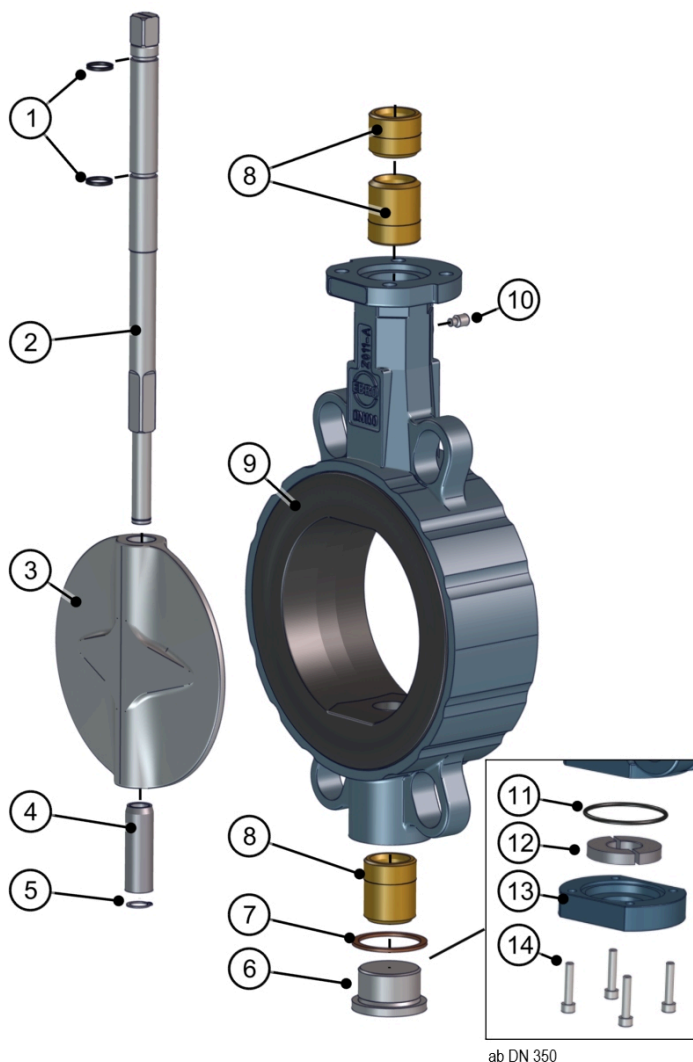
Obr. 16: Kusovník, Z011-B hriadeľ TS
