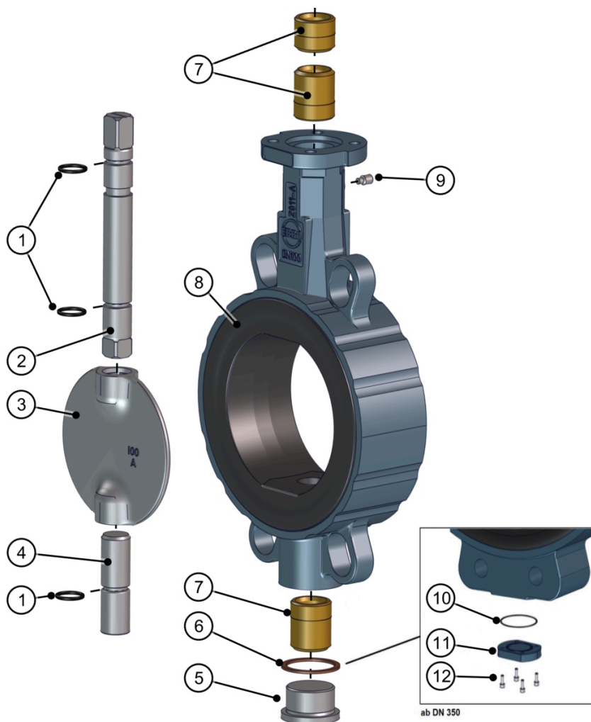
Obr. 15: Kusovník Z011-B rozdelený hriadeľ
