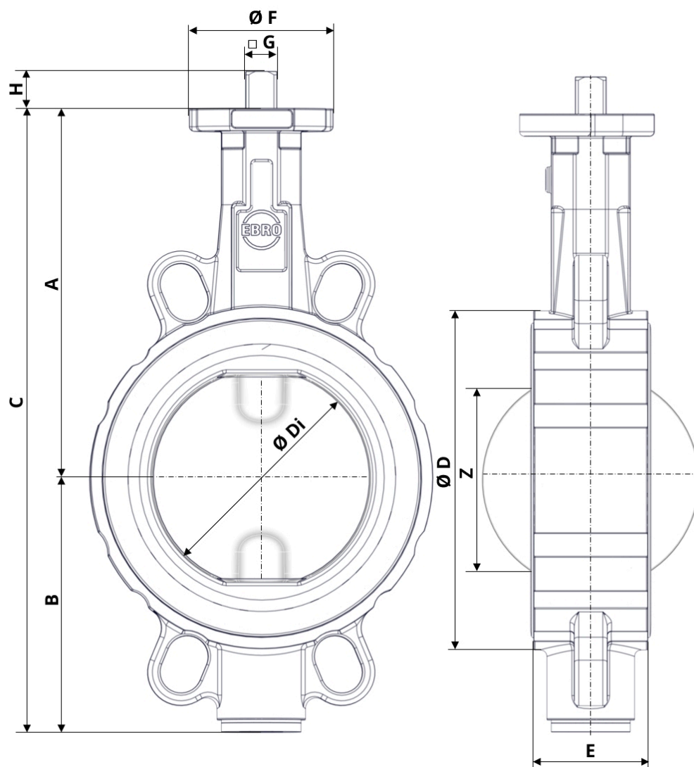
Obr. 3: Hlavné rozmery Z011-B
