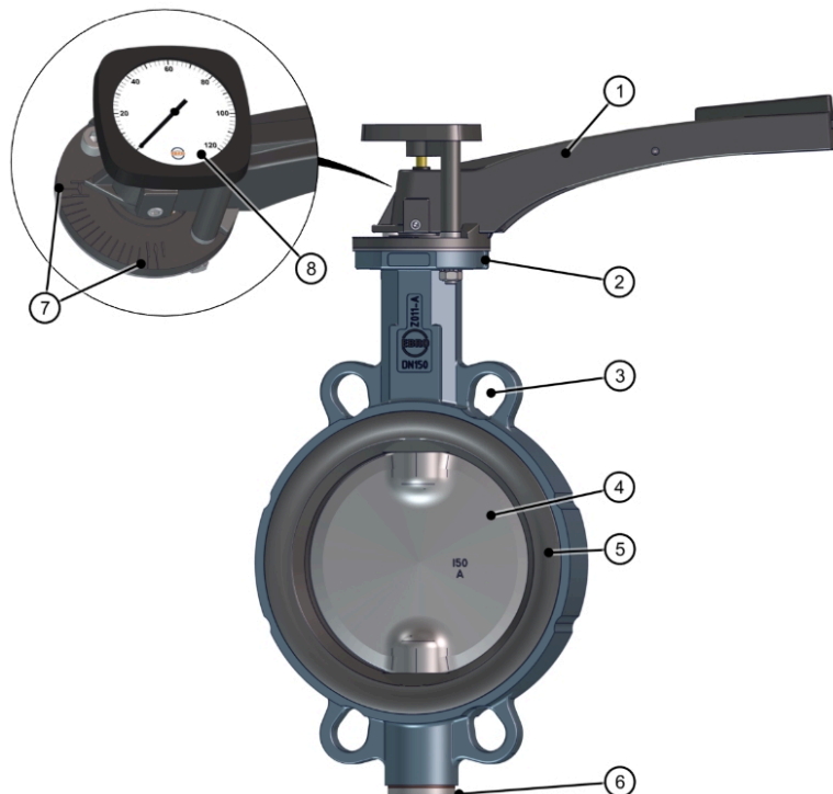
Obr. 2: Komponenty
