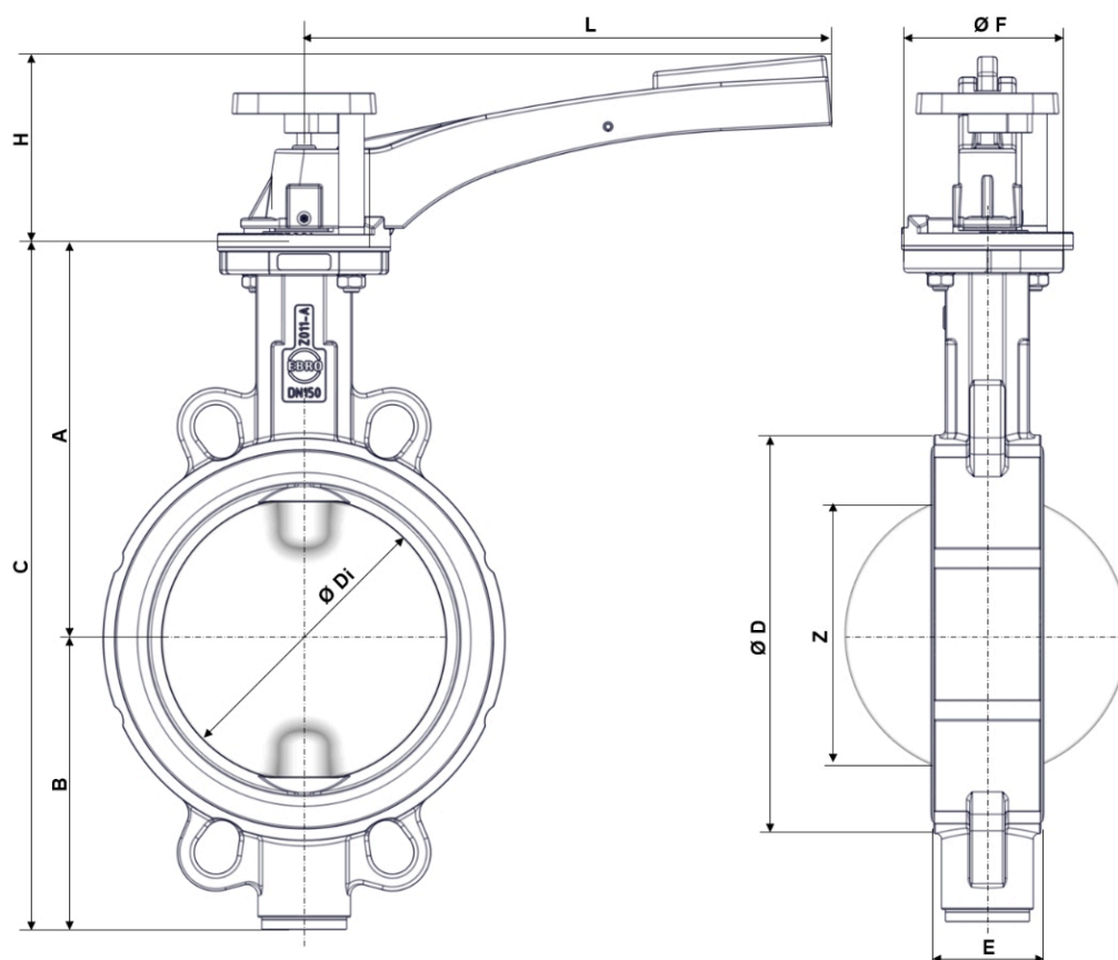
Obr. 3: Hlavné rozmery Z011-A THERM
