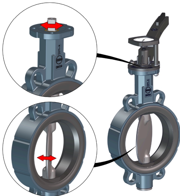
Obr. 4: Pohyblivé časti
