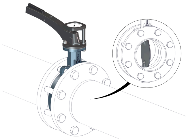
Obr. 13: Prepláchnuť potrubie
