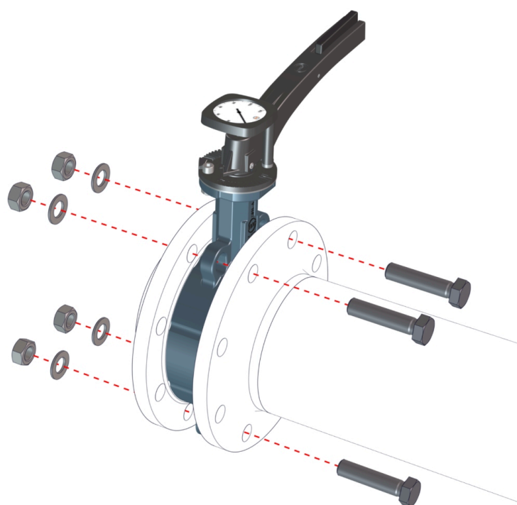
Obr. 8: Umiestnenie medziprírubovej klapky
