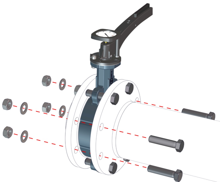
Obr. 9: Skrutkovanie medziprírubovej klapky
