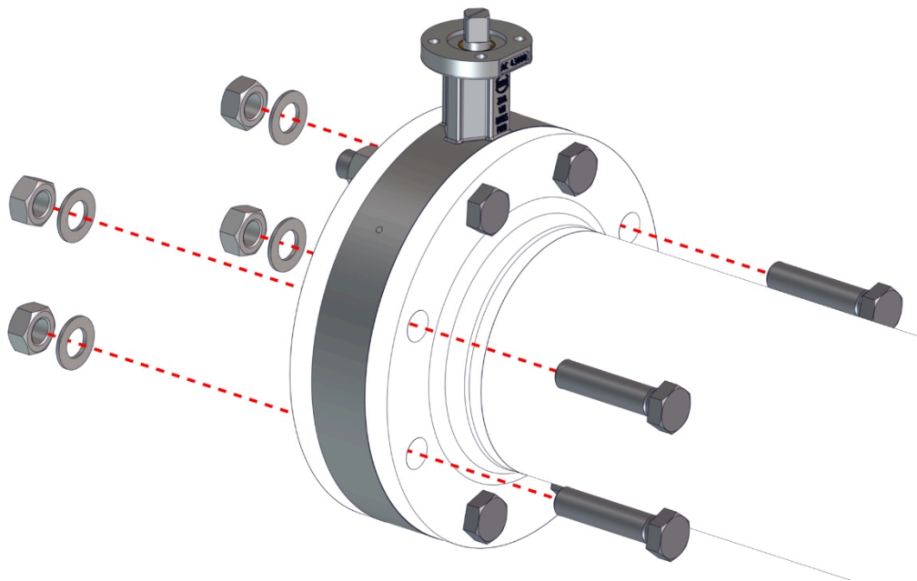
Fig. 9: Înșurubați clapeta cu flanșă completă
