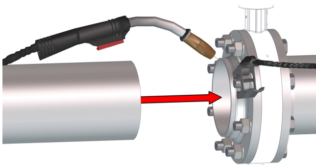
Fig. 10: Sudați țeava cu flanșa
