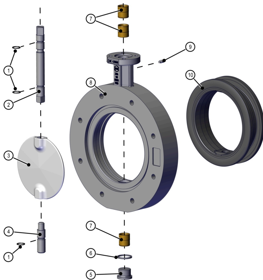
Fig. 15: Listă de componente Z014-WN
