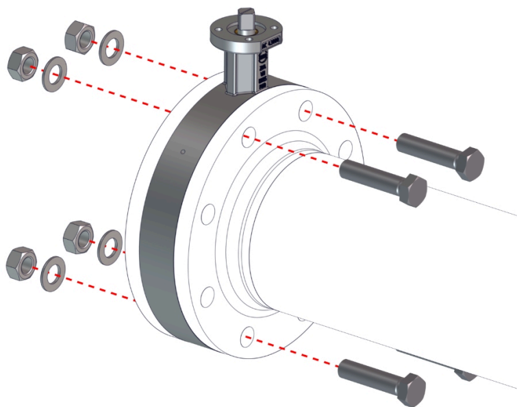
Fig. 8: Poziționați clapeta cu flanșă completă
