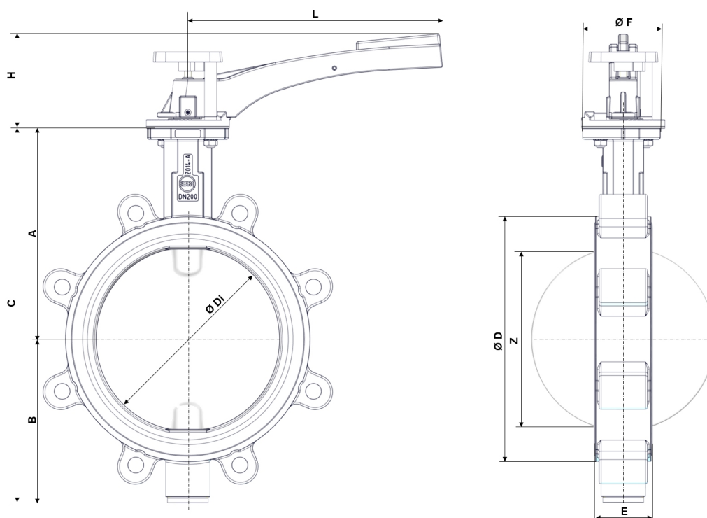
Fig. 3: Dimensiuni principale Z014-A THERM
