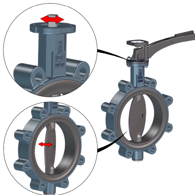
Fig. 4: Pieșele mobile
