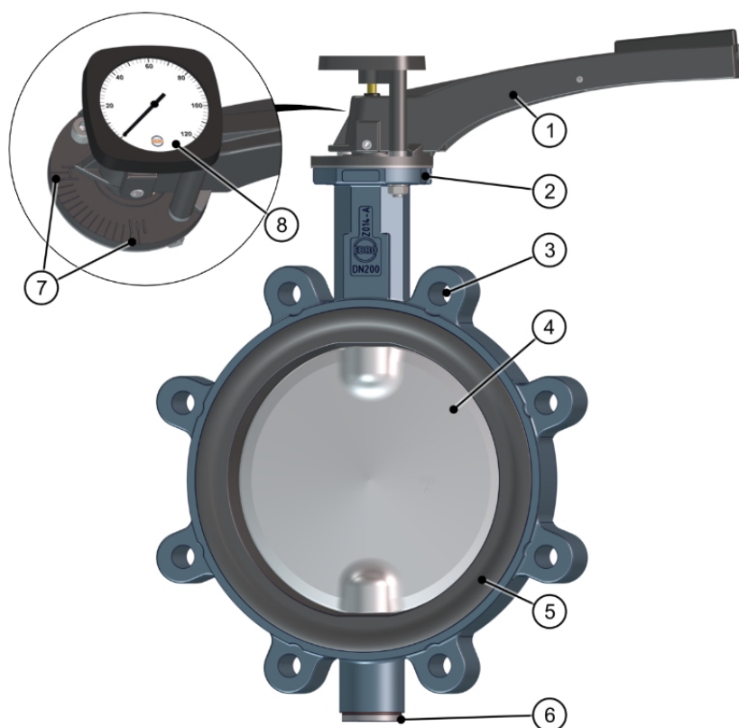
Fig. 2: Componente
