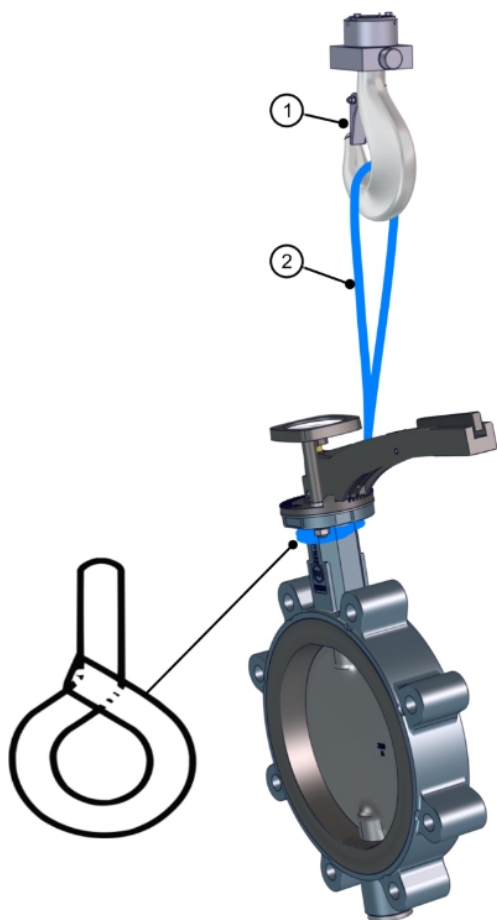
Fig. 6: Ridicarea clapetei cu flanșă cu macaraua
