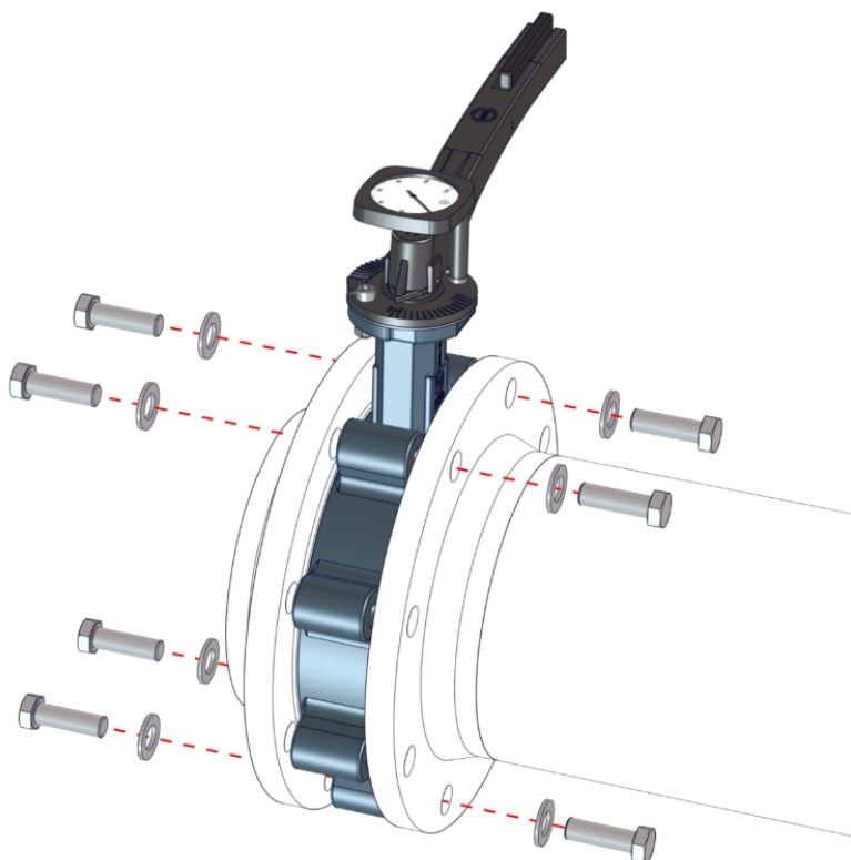
Fig. 8: Poziționați clapeta cu flanșe
