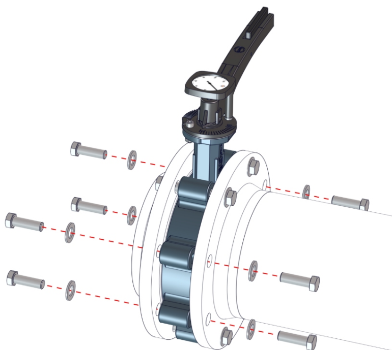
Fig. 9: Înșurubați clapeta cu flanșă
