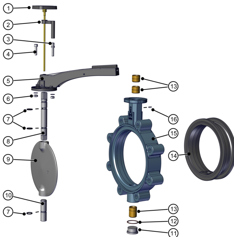
Fig. 16: Listă de componente Z014-A THERM
